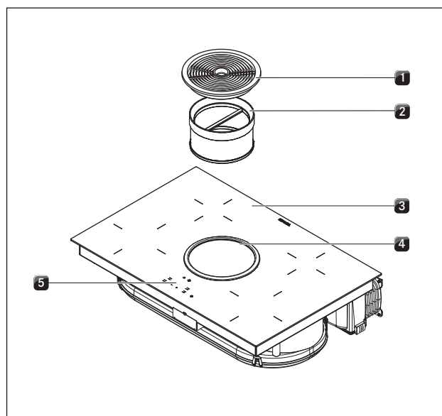
Fig. 5.1 Piano di cottura
