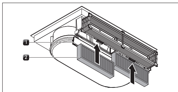
Fig. 6.16 Inserire il filtro al carbone attivo
