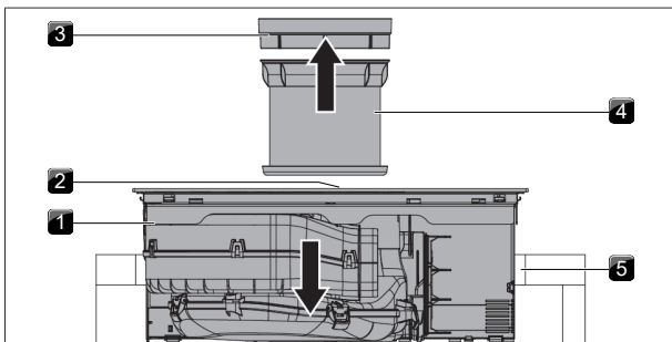
Abb. 9.16 Kochfeld einsetzen
