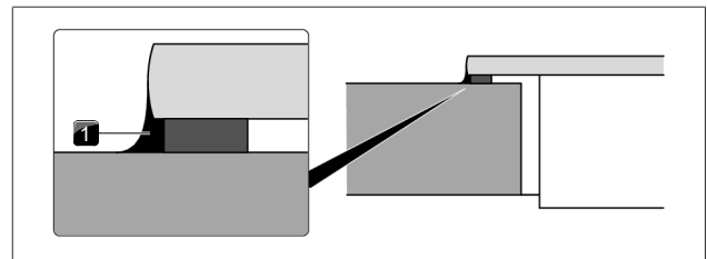
Abb. 9.31 Silikondichtmasse bei Aufsatzmontage
