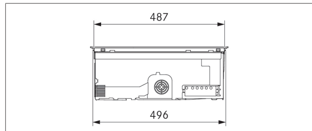
Abb. 3.3 Gerätemaße Seitenansicht
