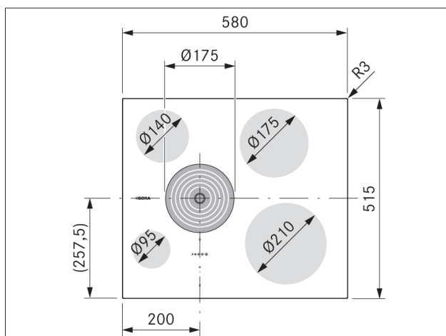
Abb. 3.1 Gerätemaße Draufsicht
