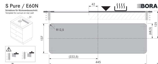
Abb. 9.9 Schablone für Rückwand-Ausschnitt
