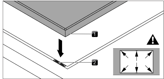
Abb. 9.18 Höhenausgleichsplatten einlegen
