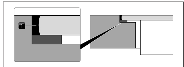
Abb. 9.32 Silikondichtmasse bei flächenbündiger Montage
