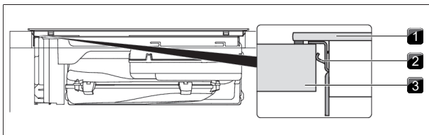
Abb. 9.17 Kochfeld befestigen
