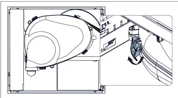
Abb. 9.21 Saugraum Verschlüsse
