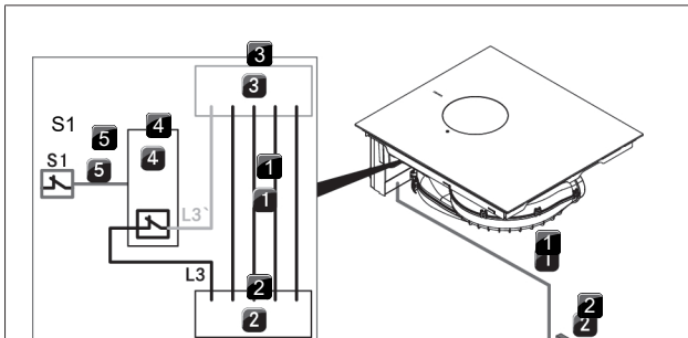
Abb. 9.27 Anschlusschema mit externen Schaltkontakten
