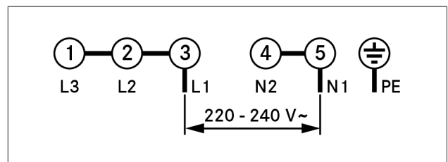
Abb. 9.25 Anschlussschema Einphasen-Anschluss
