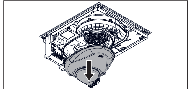
Abb. 9.22 Saugraum-Unterteil demontieren
