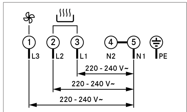
Abb. 9.23 Anschlussschema Dreiphasen-Anschluss
