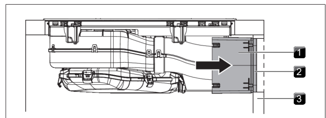
Abb. 9.20 Rückwandanschluss
