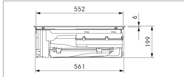
Abb. 3.2 Gerätemaße Vorderansicht
