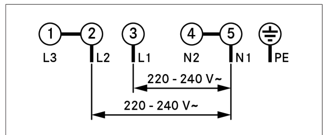
Abb. 9.24 Anschlussschema Zweiphasen-Anschluss
