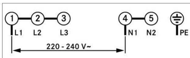
Fig. 9.24 Schema di collegamento, collegamento monofase
