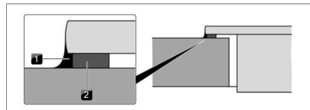
Fig. 9.14 Nastro a tenuta per montaggio in battuta
