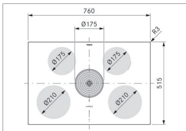
Fig. 3.1 Dimensioni apparecchio vista dall'alto
