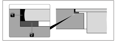
Fig. 11.18 Forseglingsstape til planlimet montage
