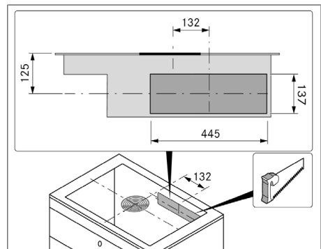
Fig. 11.11 Udskæring i bagvæggen
