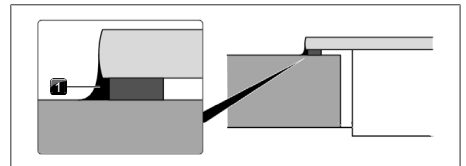
Fig. 11.35 Silikonemasse ved overflademontering
