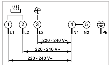
Fig. 11.27 Tilslutningsskema, 3-faset tilslutning
