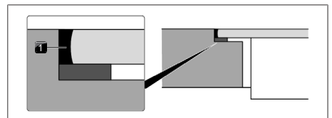
Fig. 11.36 Silikoneforseglingsmasse ved planlimet montering
