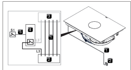
Fig. 11.26 Tilslutningsdiagram med ekstern omkøblingskontakt
