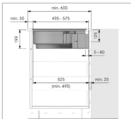
Fig. 11.13 Indbygningsmål ved recirkulationsluft, monteringsvariant A
