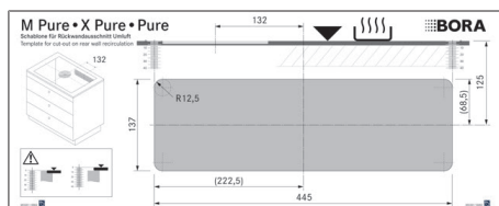
Fig. 11.12 Skabelon til udskæring i bagvæggen
