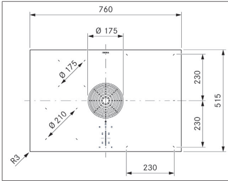
Fig. 3.4 PURMU2/R - enhedens mål set fra oven
