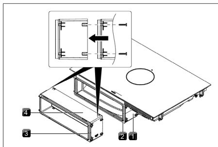
Fig. 11.15 Forlængelse af teleskopudtrækket
