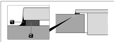
Fig. 11.17 Forseglingsstape ved overflademontage
