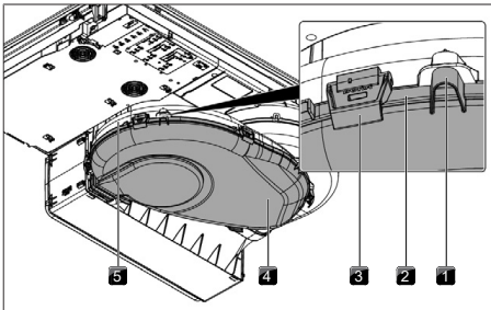
Fig. 9.3 Luftføringskabinettet
