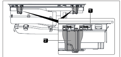
Fig. 11.19 Anbringelse af monteringsklemmer
