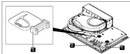
Fig. 11.30 Elektriske tilslutninger til kogepladen
