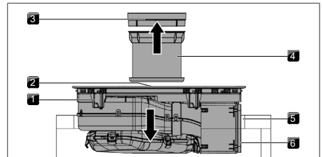
Fig. 11.20 Indsætning af kogepladen i midten
