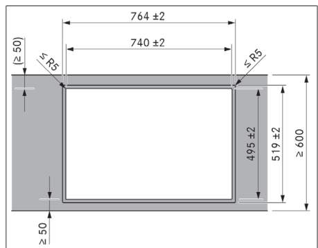
Fig. 11.5 Udskæringsmål til planimet montering
