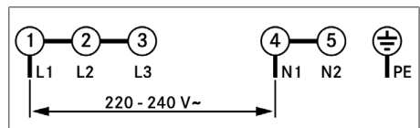
Fig. 11.28 Tilslutningsskema, 1-faset tilslutning
