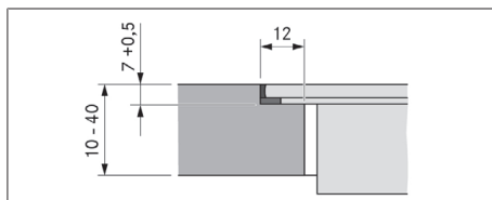
Fig. 11.6 Falsmål til planimet montering
