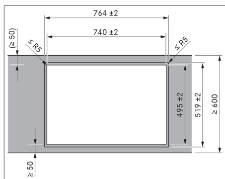
Fig. 11.5 Medidas del recorte para montaje enrasado
