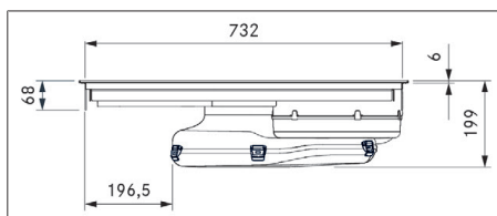
Fig. 3.2 PURMA2/R dimensiones, vista frontal
