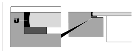
Fig. 11.36 Silicona de sellado para montaje enrasado
