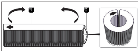
Fig. 9.7 Filtro de olores
