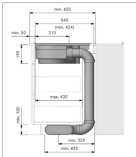
Fig. 11.9 Medidas de montaje extracción al exterior, profundidad de la encimera 600 mm
