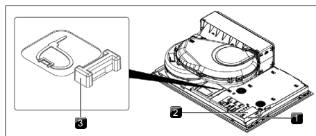
Fig. 11.30 Conexiones eléctricas de la placa de cocción
