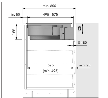
Fig. 11.13 Medidas de montaje con recirculación, variante de montaje A
