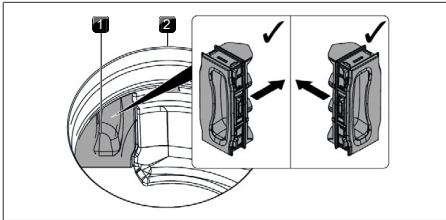
Fig. 9.10 Colocación de la trampilla para el cambio del filtro
