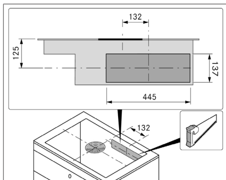
Fig. 11.11 Recorte del panel trasero
