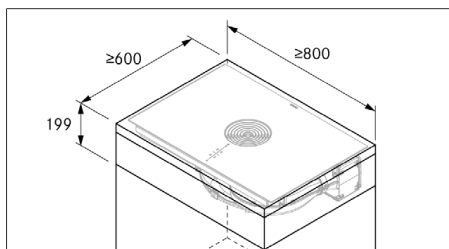
Fig. 11.4 Medidas mínimas de los muebles
