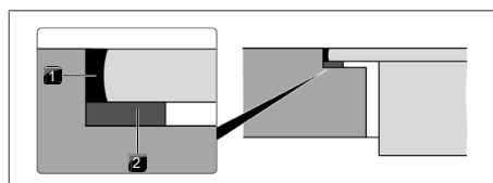
Fig. 11.18 Cinta selladora para montaje enrasado
