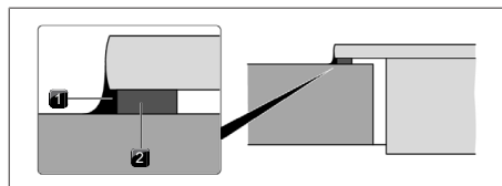
Fig. 11.17 Cinta selladora para montaje superpuesto
