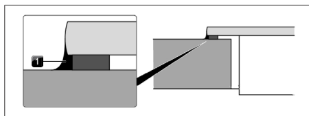
Fig. 11.35 Silicona de sellado para montaje superpuesto
