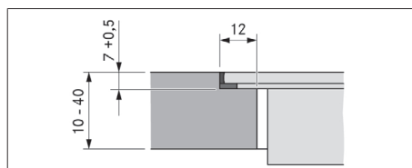
Fig. 11.6 Medida del rebaje para un montaje enrasado
