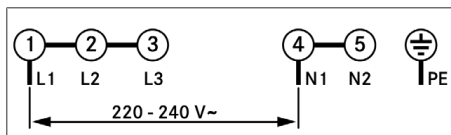
Fig. 11.28 Esquema de conexiones, conexión monofásica
