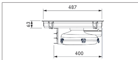
Fig. 3.3 PURMA2/R dimensiones, vista lateral
