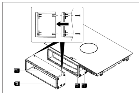
Fig. 11.15 Prolongación de la extensión telescópica
