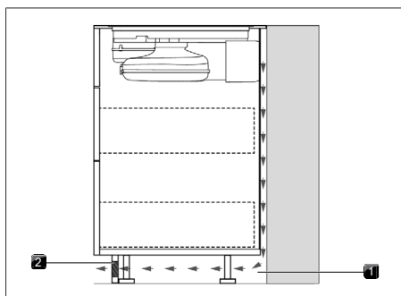
Fig. 11.10 Abertura de flujo de retorno en la zona del zócalo
