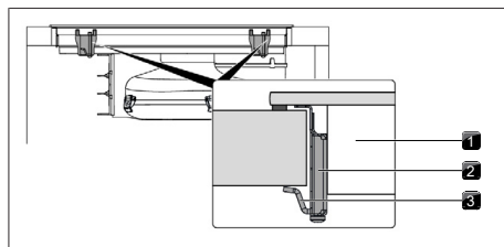
Fig. 11.23 Fijación de la placa de cocción en posición centrada
