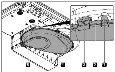
Fig. 9.3 Carcasa de conducción del aire
