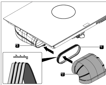
Fig. 11.24 Conexión al sistema de conductos
