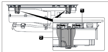
Fig. 11.19 Colocación de las abrazaderas de montaje
