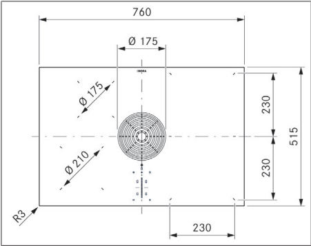
Fig. 3.4 PURMU2/R dimensiones, vista superior
