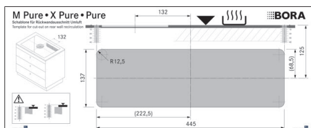
Fig. 11.12 Plantilla para el recorte del panel trasero
