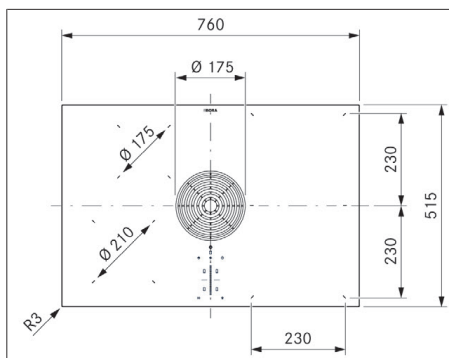
Fig. 3.1 PURMA2/R dimensiones, vista superior
