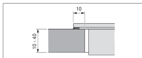
Fig. 11.8 Medida del apoyo para montaje superpuesto
