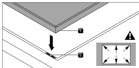
Fig. 11.21 Ubicación de placas de compensación de altura
