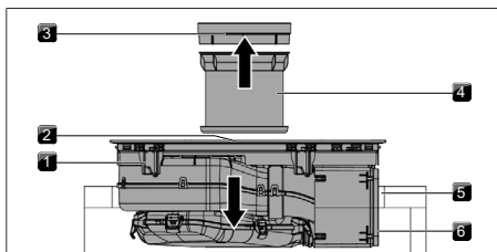
Fig. 11.20 Colocación de la placa de cocción en posición centrada
