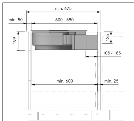
Fig. 11.14 Medidas de montaje para la variante de recirculación A, profundidad de la encimera 675 mm o más
