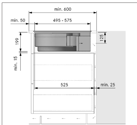
Fig. 11.16 Medidas de montaje para la variante de recirculación B, profundidad de la encimera 600 mm
