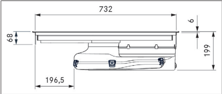
Fig. 3.5 PURMU2/R dimensiones, vista frontal
