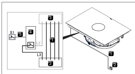
Fig. 11.26 Esquema de conexiones con contacto de conmutación externo
