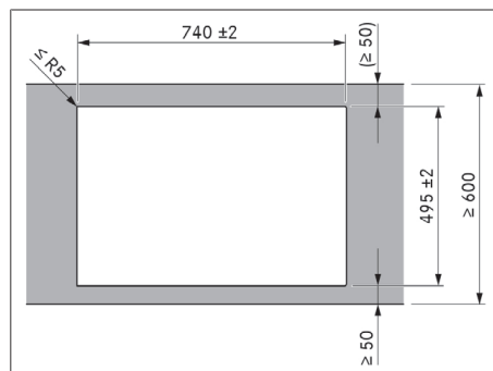
Fig. 11.7 Medidas del recorte para montaje superpuesto
