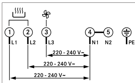
Fig. 11.27 Esquema de conexiones, conexión trifásica
