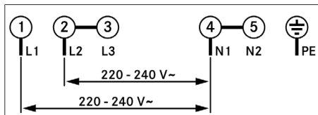
Fig. 11.29 Esquema de conexiones, conexión bifásica
