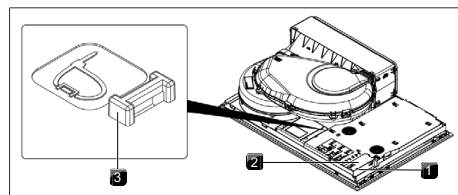
Fig. 11.30 Raccordements électriques de la table de cuisson
