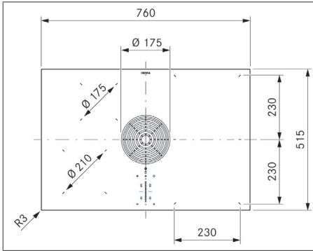
Fig. 3.4 Dimensions PURMU2/R - Vue de dessus
