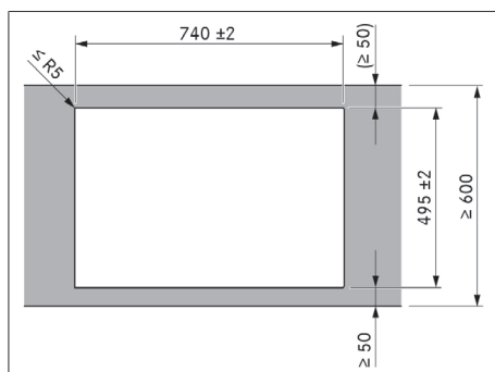
Fig. 11.7 Dimensions de découpe pour montage en saillie
