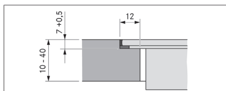
Fig. 11.6 Dimension de rainure pour montage affleurant
