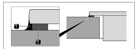
Fig. 11.17 Ruban d'étanchéité pour montage en saillie
