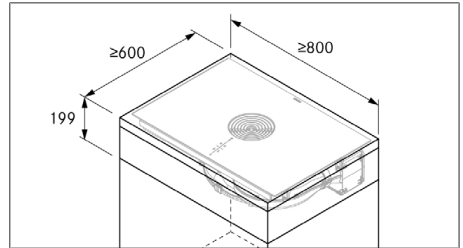
Fig. 11.4 Dimensions minimales du meuble
