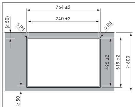
Fig. 11.5 Dimensions de découpe pour montage affleurant
