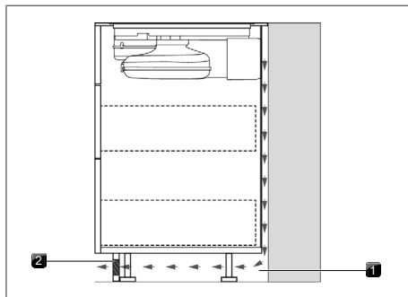
Fig. 11.10 Apertura di sfogo nell'area dello zoccolo
