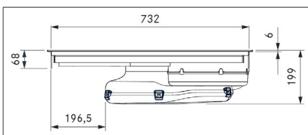
Fig. 3.2 PURMA2/R dimensioni apparecchio vista frontale
