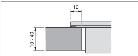
Fig. 11.8 Misura d'appoggio per montaggio in battuta
