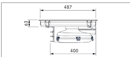
Fig. 3.3 PURMA2/R dimensioni apparecchio vista laterale
