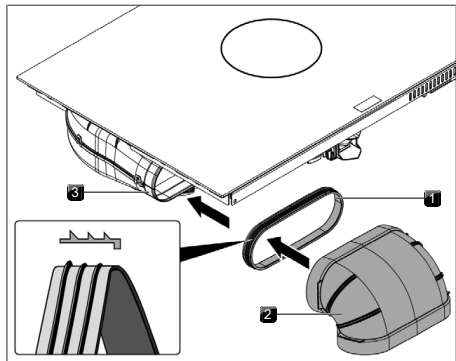
Fig. 11.24 Connessione al sistema di canali
