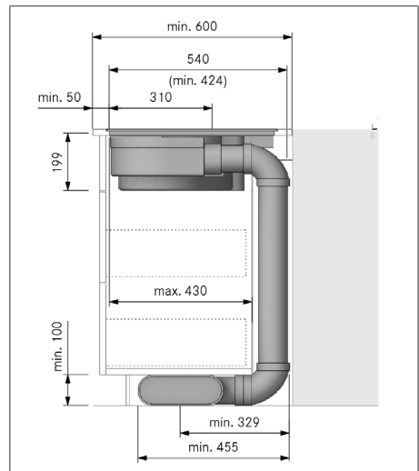
Fig. 11.9 Dimensioni di montaggio con sistema aspirante, profondità piano di lavoro 600 mm
