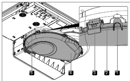
Fig. 9.3 Alloggiamento condotta aria
