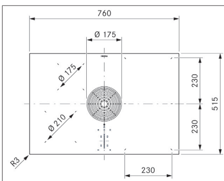
Fig. 3.1 PURMA2/R dimensioni apparecchio vista dall'alto
