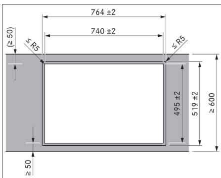
Fig. 11.5 Dimensioni intaglio per montaggio a filo
