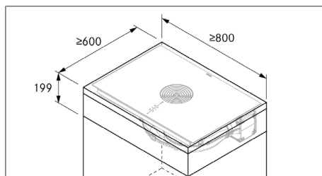
Fig. 11.4 Dimensioni minime mobile
