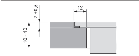
Fig. 11.6 Dimensioni dell'incassatura per montaggio a filo piano
