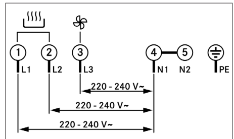
Afb. 11.27 Aansluitschema 3-faseaansluiting
