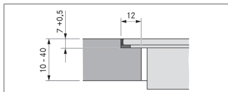
Afb. 11.6 Voegmaat voor vlinkinbouw
