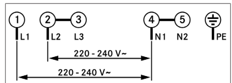
Afb. 11.29 Aansluitschema 2-faseaansluiting
