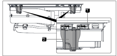
Afb. 11.19 Montageklemmen aanbrengen
