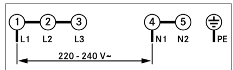
Afb. 11.28 Aansluitschema 1-faseaansluiting
