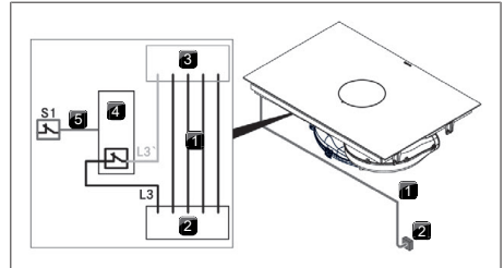
Afb. 11.26 Aansluitschema met extern schakelcontact
