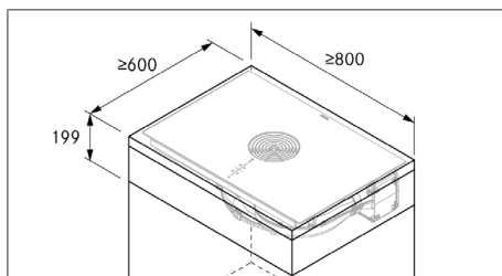
Fig. 11.4 Møbel-minstemål
