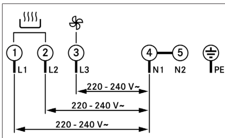
Fig. 11.27 Koblingsskjema 3-fase-tilkobling
