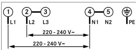
Fig. 11.29 Koblingsskjema 2-fase-tilkobling
