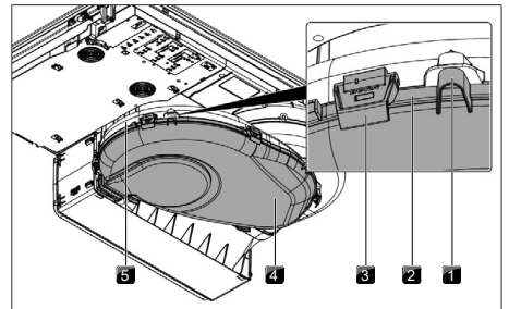
Fig. 9.3 Luftføringsapparatet
