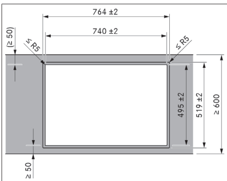
Fig. 11.5 Utskjæringsmål for planlimt montering
