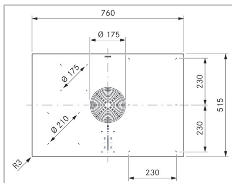
Fig. 3.4 PURMU2/R apparatdimensjoner sett ovenfra
