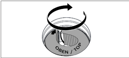
Fig. 9.9 Plassere luktfileret i sluttposisjonen
