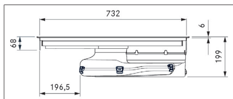
Fig. 3.5 PURMU2/R apparatdimensjoner sett forfra
