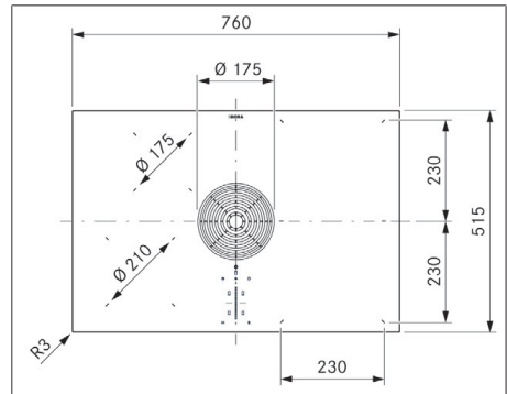
Fig. 3.1 PURMA2/R apparatdimensjoner sett ovenfra
