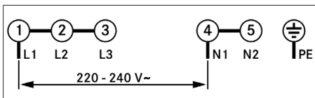
Fig. 11.28 Koblingsskjema 1-fase-tilkobling
