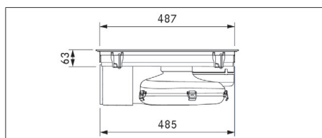
Fig. 3.6 PURMU2/R apparatdimensjoner sett fra siden
