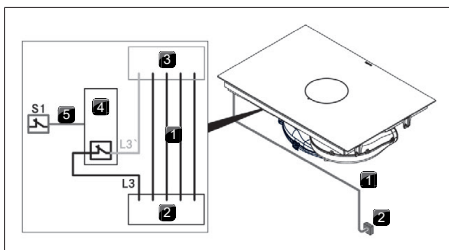
Fig. 11.26 Koblingsskjema med ekstern bryterkontakt
