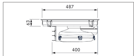
Fig. 3.3 PURMA2/R apparatdimensjoner sett fra siden
