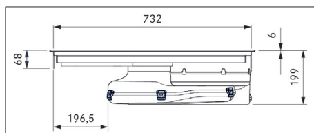
Fig. 3.5 PURMU2/R dimensões do aparelho vista frontal
