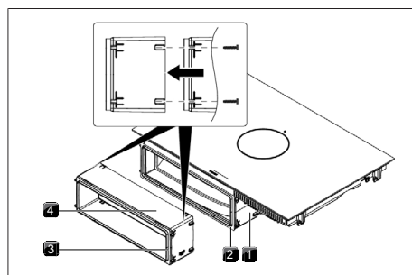
Fig. 11.15 Extensão da guia telescópica
