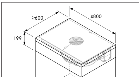
Fig. 11.4 Dimensões mínimas do móvel
