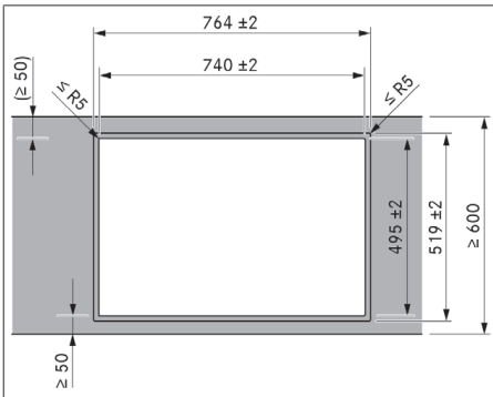
Fig. 11.5 Medidas de recorte para montagem à face
