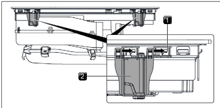
Fig. 11.19 Instalar grampos de montagem
