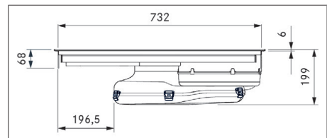
Fig. 3.2 PURMA2/R dimensões do aparelho vista frontal
