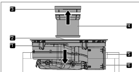
Fig. 11.20 Colocar a placa de cozinhar centrada
