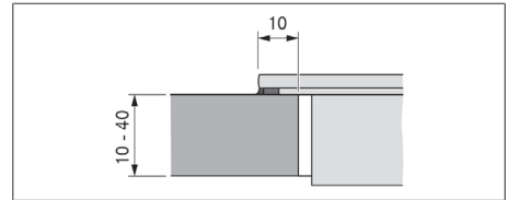
Fig. 11.8 Medida do apoio para montagem por sobreposição
