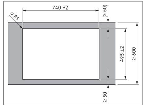
Fig. 11.7 Medidas de recorte para montagem por sobreposição
