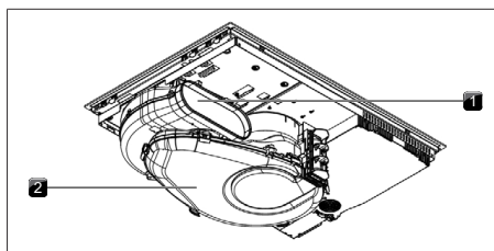
Fig. 4.2 Vista traseira da versão de extração de ar
