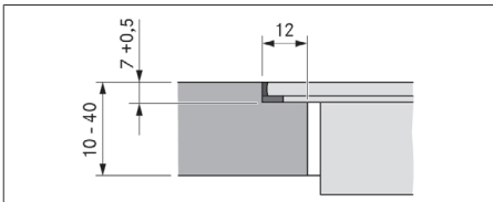
Fig. 11.6 Medida de recesso para montagem à face
