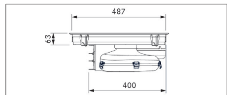
Fig. 3.3 PURMA2/R dimensões do aparelho vista lateral
