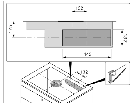
Fig. 11.11 Recorte do painel traseiro
