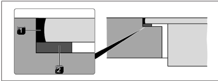
Fig. 11.18 Cinta vedante na montagem à face
