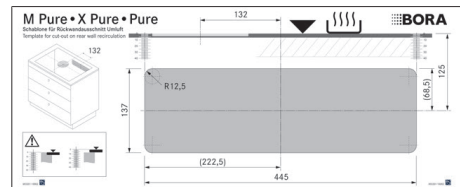
Fig. 11.12 Molde para o recorte do painel traseiro
