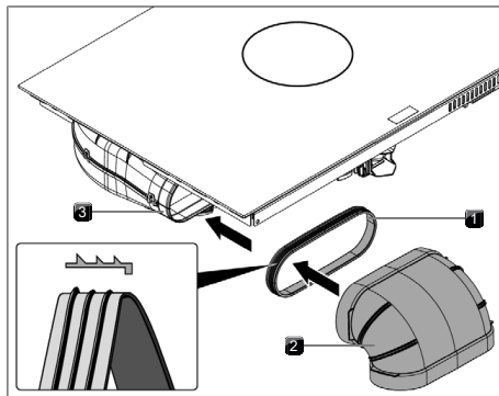
Fig. 11.24 Ligação ao sistema de condutas
