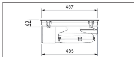
Fig. 3.6 PURMU2/R dimensões do aparelho vista lateral
