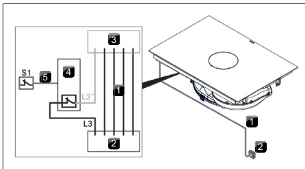
Fig. 11.26 Esquema de ligação com comutador externo
