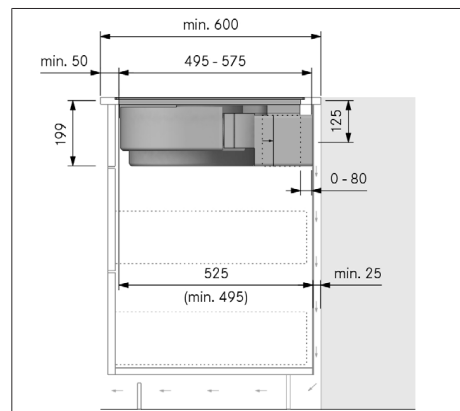
Fig. 11.13 Medidas de instalação para a recirculação de ar, variante de montagem A
