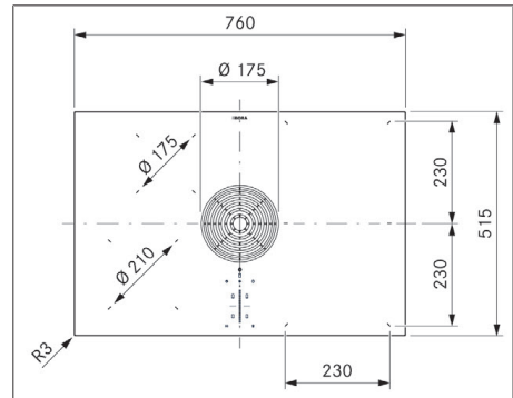
Fig. 3.1 PURMA2/R dimensões do aparelho vista de cima
