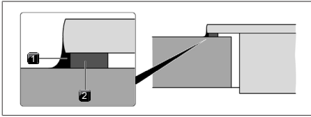
Fig. 11.17 Cinta vedante para montagem por sobreposição
