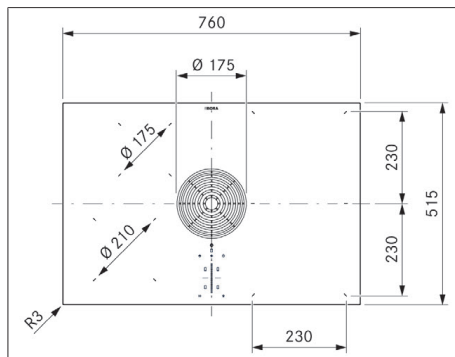
Fig. 3.4 PURMU2/R dimensões do aparelho vista de cima
