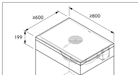
obr. 11.4 Minimální rozměry nábytku
