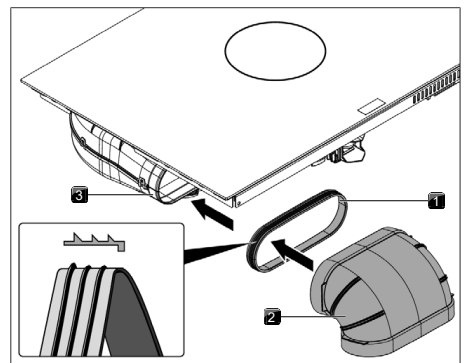
obr. 11.24 Připojení systému odtahových potrubí
