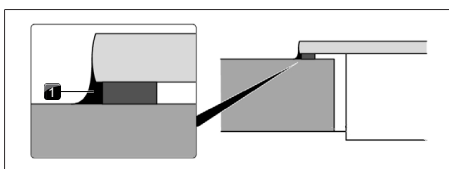
obr. 11.35 Silikonová těsnicí hmota při montáži na povrch
