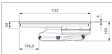
obr. 3.2 Rozměry spotřebiče PURA2/R – pohled zepředu
