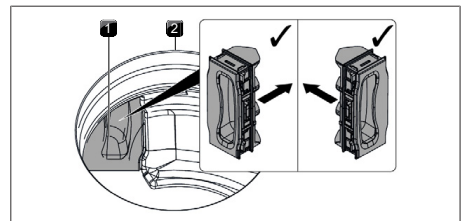
obr. 9.10 Nasazení výměnné klapky filtru
