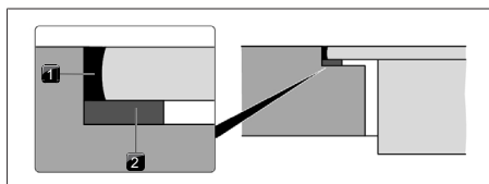
obr. 11.18 Těsnicí páska při plošně zarovnané montáži
