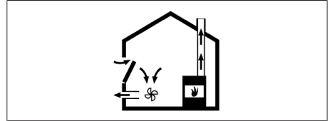
obr. 11.2 Montáž odtahu ven – správná
