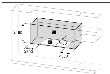
obr. 11.3 Požadovaný volný prostor
