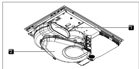
obr. 4.2 Pohled zezadu na variantu odtahu ven
