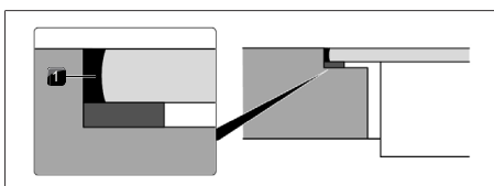
obr. 11.36 Silikonová těsnicí hmota při plošně zarovnané montáži
