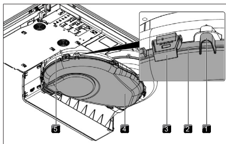
obr. 9.3 Skříň ventilace
