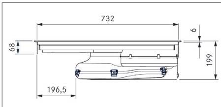
obr. 3.5 Rozměry spotřebiče PURU2/R – pohled zepředu
