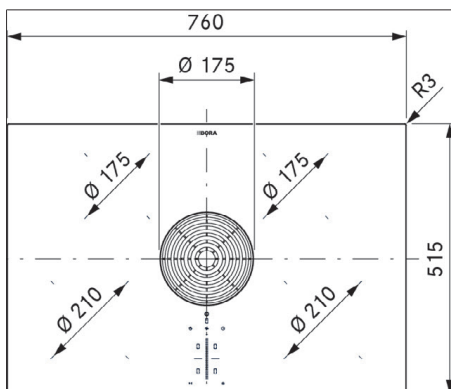
obr. 3.1 Rozměry spotřebiče PURA2/R – pohled shora
