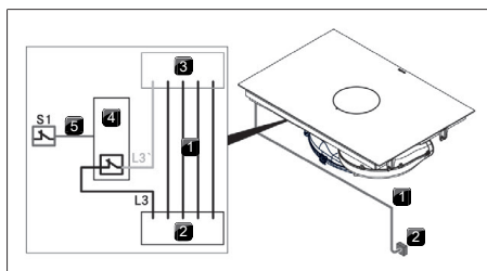
obr. 11.26 Schéma zapojení s externím spínacím kontaktem
