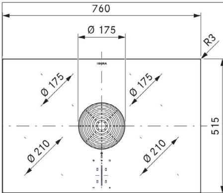
obr. 3.4 Rozměry spotřebiče PURU2/R – pohled shora
