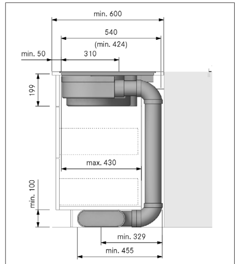
obr. 11.9 Rozměry montáže při odtaň ven, hloubka pracovní desky 600 mm
