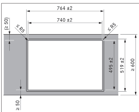
obr. 11.5 Rozměry výřezu pro plošně zarovnanou montáž
