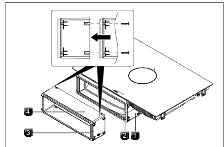
obr. 11.15 Nastavení teleskopického výsuvu
