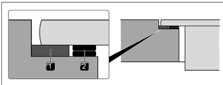
obr. 11.22 Podložky k nastavení výšky
