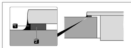
obr. 11.17 Těsnicí páska při montáži na povrch
