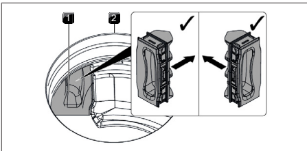
Abb. 9.10 Filterwechselklappe einsetzen
