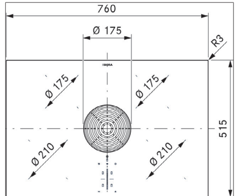
Abb. 3.1 PURA2/R Gerätemaße Draufsicht
