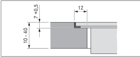
Abb. 11.6 Falzmaß für flächenbündige Montage
