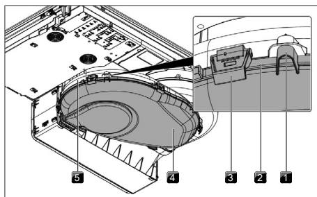
Abb. 9.3 Luftführungsgehäuse
