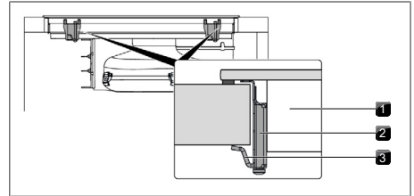
Abb. 11.23 Kochfeld mittig befestigen
