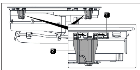
Abb. 11.19 Montageklammern anbringen
