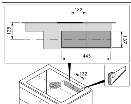
Abb. 11.11 Rückwand-Ausschnitt
