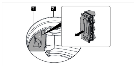
Abb. 9.4 Filterwechselklappe entfernen
