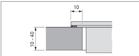
Abb. 11.8 Auflagemaß für Aufsatzmontage
