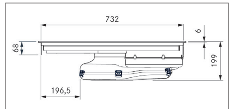
Abb. 3.2 PURA2/R Gerätemaße Vorderansicht
