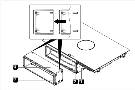
Fig. 11.15 Prolongación de la extensión telescópica
