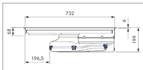
Fig. 3.5 Medidas del aparato PURU2/R, vista frontal
