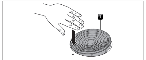
Fig. 9.1 Retirar la tobera de entrada
