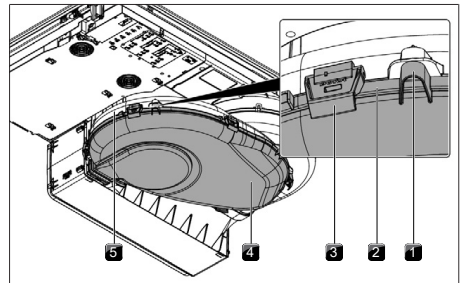
Fig. 9.3 Carcasa de conducción del aire
