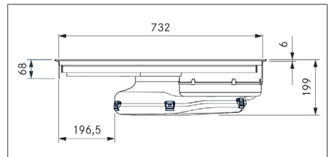
Fig. 3.2 Medidas del aparato PURA2/R, vista frontal
