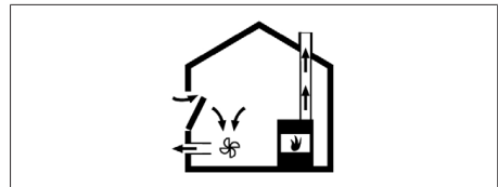
Fig. 11.2 Instalación de la extracción al exterior - correcta
