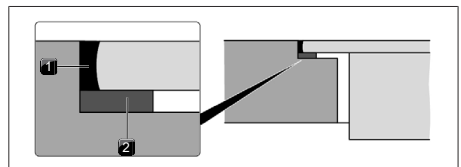
Fig. 11.18 Cinta selladora para montaje enrasado
