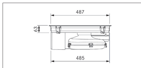
Fig. 3.6 Medidas del aparato PURU2/R, vista lateral
