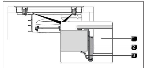
Fig. 11.23 Fijación de la placa de cocción en posición centrada
