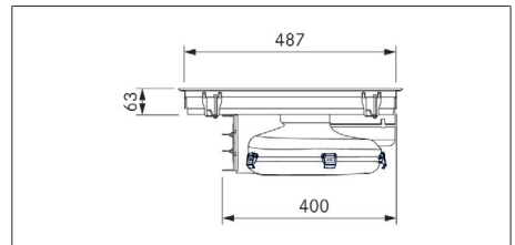
Fig. 3.3 Medidas del aparato PURA2/R, vista lateral
