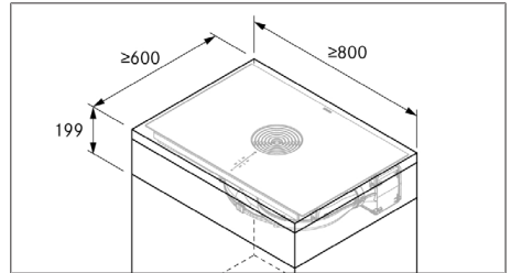
Fig. 11.4 Medidas mínimas de los muebles
