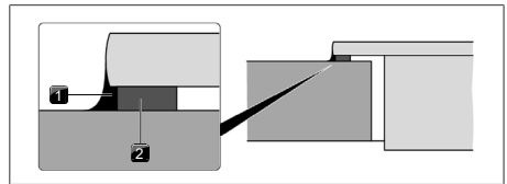
Fig. 11.17 Cinta selladora para montaje superpuesto
