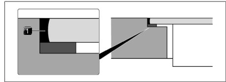
Fig. 11.36 Silicona de sellado para montaje enrasado
