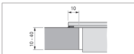
Fig. 11.8 Medida del apoyo para montaje superpuesto
