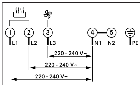
Fig. 11.27 Esquema de conexiones, conexión trifásica
