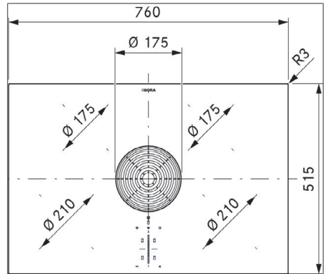
Fig. 3.1 Medidas del aparato PURA2/R, vista superior
