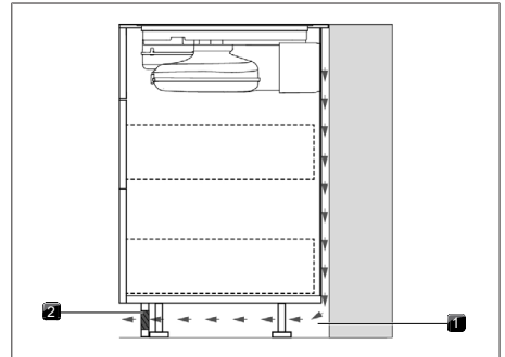
Fig. 11.10 Abertura de flujo de retorno en la zona del zócalo
