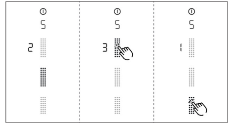
Fig. 8.6 Opción de menú 5: Velocidad de reacción
