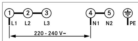
Fig. 11.28 Esquema de conexiones, conexión monofásica
