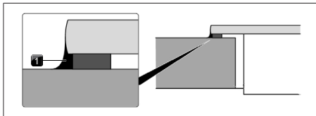
Fig. 11.35 Silicona de sellado para montaje superpuesto
