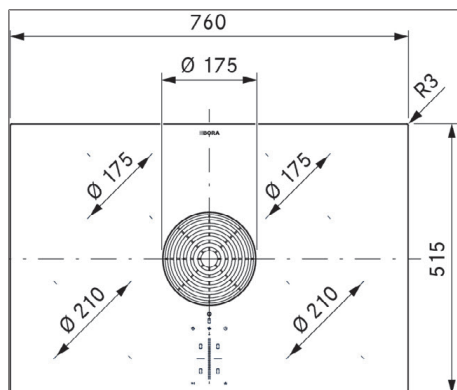
Fig. 3.4 Medidas del aparato PURU2/R, vista superior
