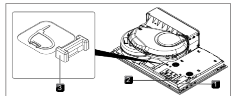
Kuva 11.30 Keittotason sähköliitäntä
