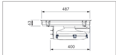
Kuva 3.3 Laitemitat PURA2/R sivukuva
