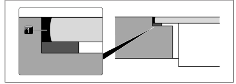
Kuva 11.36 Silikonitiivistysmassa uppoasennuksessa
