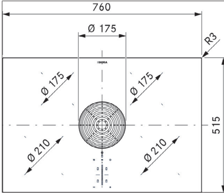
Kuva 3.4 Laitemitat PURU2/R kuva ylhäältä
