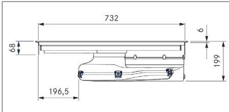
Kuva 3.5 Laitemitat PURU2/R kuva edestä
