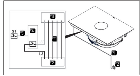
Kuva 11.26 Liittätäkaavio, ulkoinen kytkin
