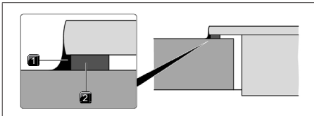
Kuva 11.17 Tiivistenauha pinta-asennuksessa
