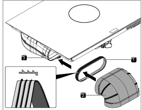
Kuva 11.24 Liittäminen kanavajärjestelmään
