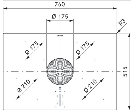
Kuva 3.1 Laitemitat PURA2/R kuva ylhäältä
