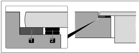
Kuva 11.22 Korkeussäätölevyt
