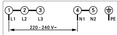
Kuva 11.28 Liittätäkaavio - 1-vaiheiliitäntä
