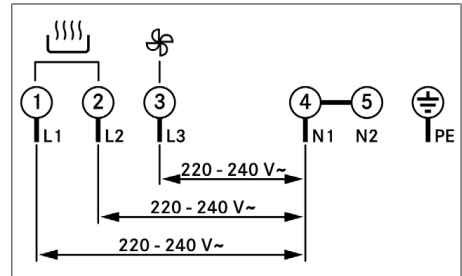
Kuva 11.27 Liittätäkaavio - 3-vaiheiliitäntä
