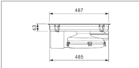
Kuva 3.6 Laitemitat PURU2/R sivukuva
