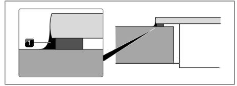
Kuva 11.35 Silikonitiivistysmassa pinta-asennuksessa
