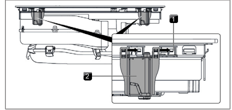
Kuva 11.19 Kiinnittimien kiinnittäminen
