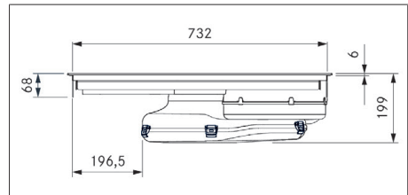
Kuva 3.2 Laitemitat PURA2/R kuva edestä
