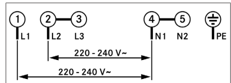
Kuva 11.29 Liittätäkaavio - 2-vaiheiliitäntä
