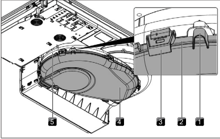
Kuva 9.3 Ilmanohjauksetelo
