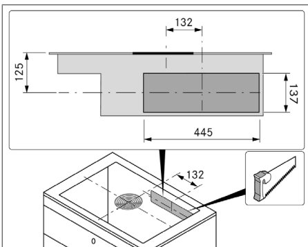
Fig. 11.11 Sezione parete posteriore
