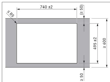
Fig. 11.7 Dimensioni intaglio per montaggio in battuta
