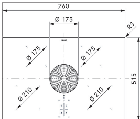
Fig. 3.4 PURU2/R dimensioni apparecchio vista dall'alto
