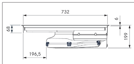
Fig. 3.5 PURU2/R dimensioni apparecchio vista frontale
