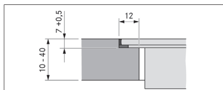
Fig. 11.6 Dimensioni dell'incassatura per montaggio a filo piano
