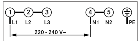
Fig. 11.28 Schema di collegamento, collegamento monofase
