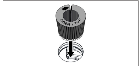
Fig. 9.8 Inserire il filtro antiodori nell'apertura di aspirazione
