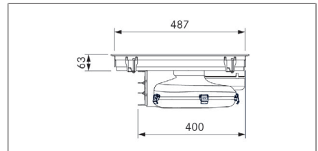
Fig. 3.3 PURA2/R dimensioni apparecchio vista laterale
