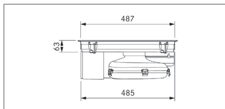
Fig. 3.6 PURU2/R dimensioni apparecchio vista laterale
