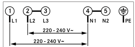
Fig. 11.29 Schema di collegamento, collegamento bifase
