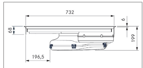
Fig. 3.2 PURA2/R dimensioni apparecchio vista frontale
