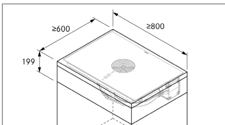
Fig. 11.4 Dimensioni minime mobile
