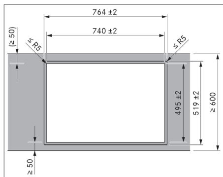
Fig. 11.5 Dimensioni intaglio per montaggio a filo
