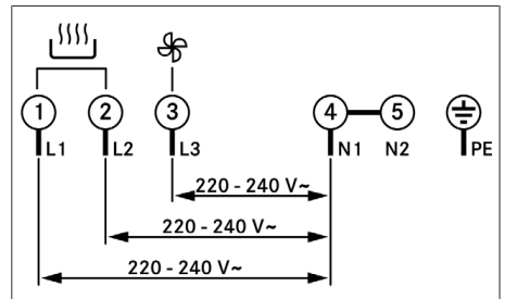
Fig. 11.27 Schema di collegamento, collegamento trifase
