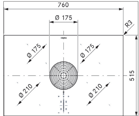
Fig. 3.1 PURA2/R dimensioni apparecchio vista dall'alto
