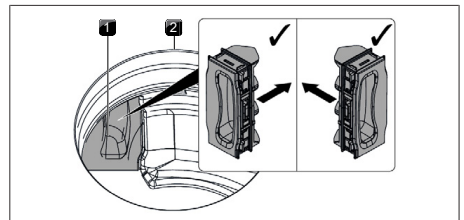
Fig. 9.10 Inserire la valvola di sostituzione del filtro
