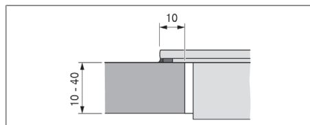
Fig. 11.8 Misura d'appoggio per montaggio in battuta
