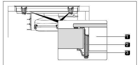
Afb. 11.23 Centrale bevestiging kookveld
