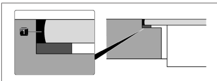
Afb. 11.36 Siliconenkit bij vlakbouw
