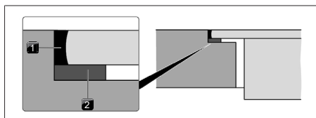
Afb. 11.18 Afdichtingsband bij vlakinbouw
