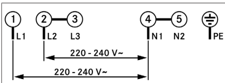
Afb. 11.29 Aansluitschema 2-faseaansluiting
