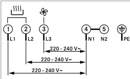
Afb. 11.27 Aansluitschema 3-faseaansluiting
