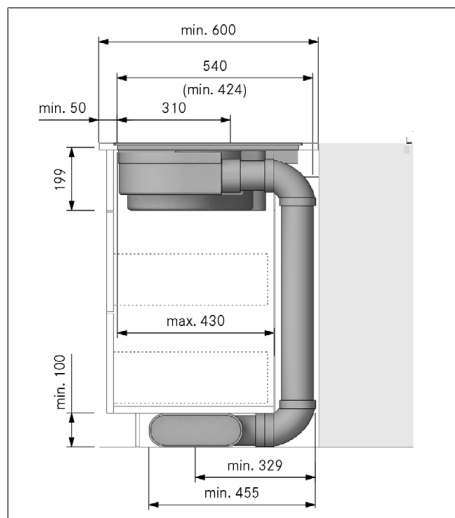
Afb. 11.9 Inbouwmaten luchtafvoer, werkbladdiepte 600 mm
