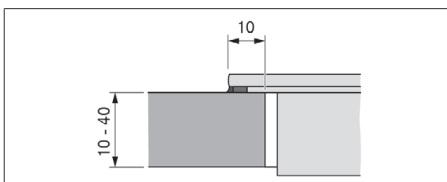
Afb. 11.8 Oplegmaat voor opbouwmontage
