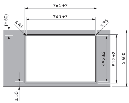
Afb. 11.5 Uitsparingsafmetingen in geval van vlakinbouw
