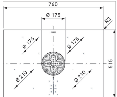
Afb. 3.1 PURA2/R apparaatafmetingen bovenaanzicht
