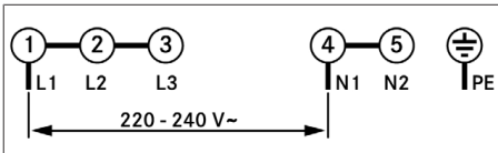
Afb. 11.28 Aansluitschema 1-faseaansluiting
