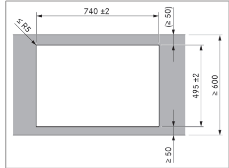
Rys. 11.7 Wymiary wycięcia dla montażu elementu z uskokiem
