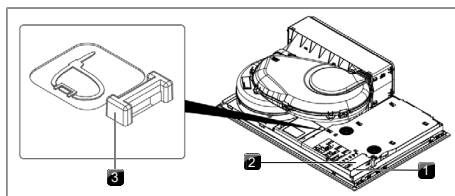
Rys. 11.30 Przyłącza elektryczne płyty grzewczej
