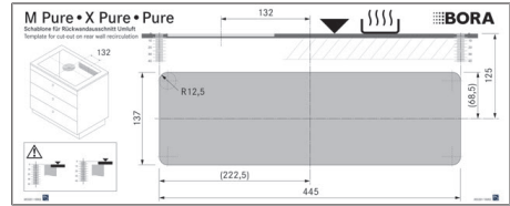
Rys. 11.12 Szablon do wycięcia ściany tylnej
