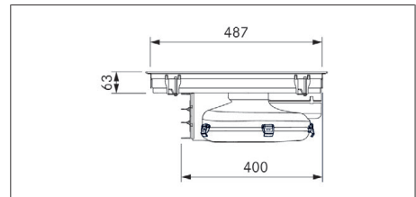
Rys. 3.3 PURA2/R Wymiary urządzenia - widok z boku
