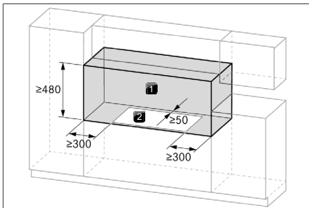
Rys. 11.3 Wymagane odstępy
