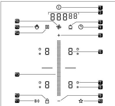
Rys. 4.4 Panel sterowania
