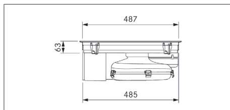
Rys. 3.6 PURU2/R Wymiary urządzenia – widok z boku
