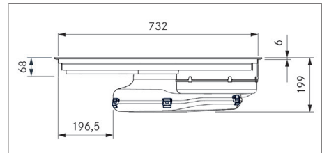
Rys. 3.2 PURA2/R Wymiary urządzenia - widok z przodu
