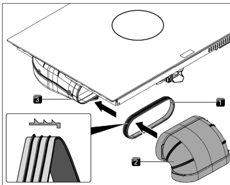
Rys. 11.24 Podłączenie do systemu kanałów
