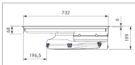
Rys. 3.5 PURU2/R Wymiary urządzenia – widok z przodu
