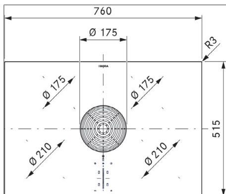
Rys. 3.4 PURU2/R Wymiary urządzenia – widok z góry
