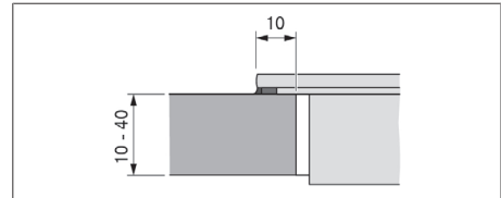
Rys. 11.8 Wymiary podparcia dla montażu elementu z uskokiem
