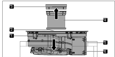
Rys. 11.20 Centralne ustawianie płyty grzewczej
