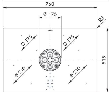
Rys. 3.1 PURA2/R Wymiary urządzenia - widok z góry
