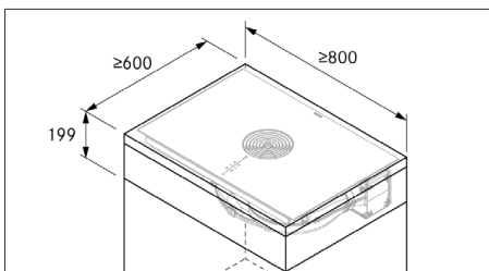
Rys. 11.4 Minimalne wymiary mebli
