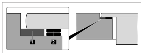
Rys. 11.22 Podkładki wyrównujące
