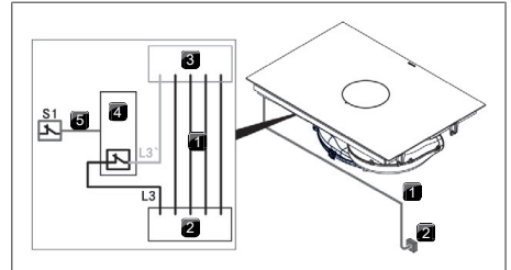
Rys. 11.26 Schemat podłączenia z zewnętrznym stykiem przełączającym
