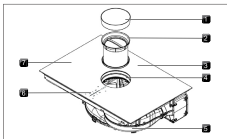
Rys. 4.1 Budowa
