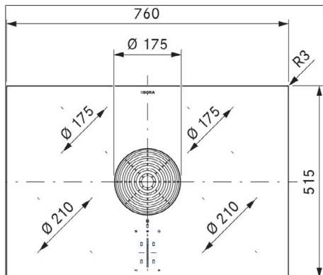
Fig. 3.4 PURU2/R dimensões do aparelho vista de cima
