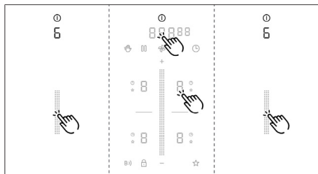
Fig. 8.7 Opção de menu 6: Teste dos LED
