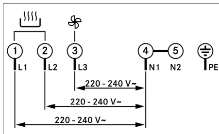
Fig. 11.27 Esquema de ligações trifásico
