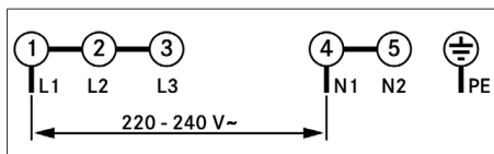
Fig. 11.28 Esquema de ligações monofásico
