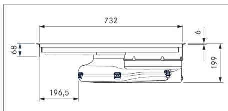
Fig. 3.5 PURU2/R dimensões do aparelho vista frontal
