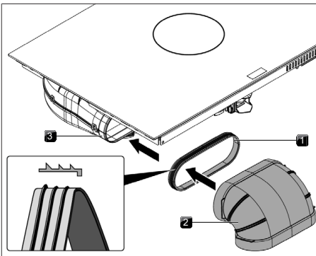
Fig. 11.24 Ligação ao sistema de condutas
