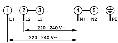
Fig. 11.29 Esquema de ligações bifásico
