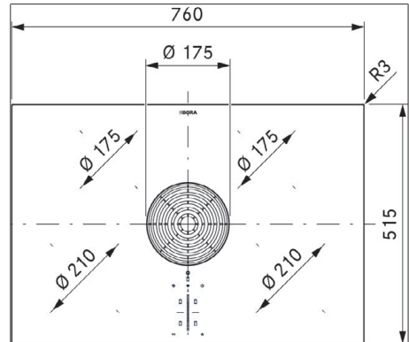
Fig. 3.1 PURA2/R dimensões do aparelho vista de cima
