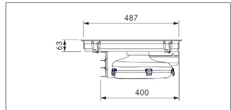
Fig. 3.3 PURA2/R dimensões do aparelho vista lateral
