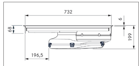
Fig. 3.2 PURA2/R dimensões do aparelho vista frontal
