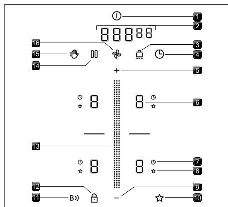
Fig. 4.4 Painel de comando
