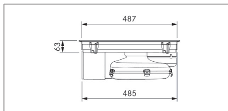
Fig. 3.6 PURU2/R dimensões do aparelho vista lateral
