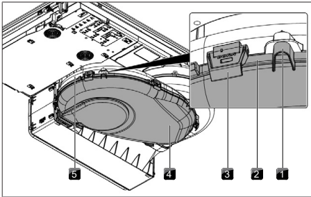
Fig. 9.3 Carcaça de condução do ar
