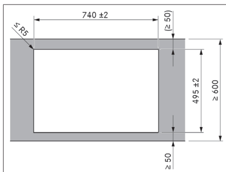
Fig. 11.7 Medidas de recorte para montagem por sobreposição
