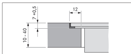
Fig. 11.6 Medida de recesso para montagem à face
