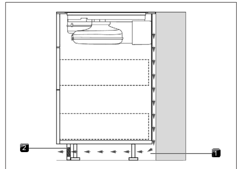
Fig. 11.10 Abertura de retorno na zona de rodapé
