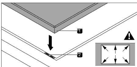
Fig. 11.21 Posicionamento e placas de compensação de altura
