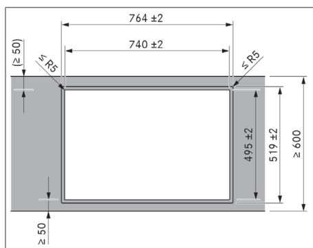
Fig. 11.5 Medidas de recorte para montagem à face
