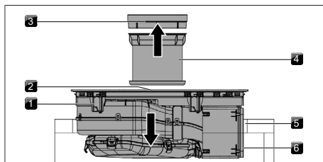
Fig. 11.20 Colocar a placa de cozinhar centrada
