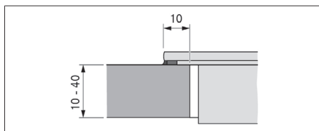
Fig. 11.8 Medida do apoio para montagem por sobreposição
