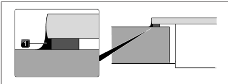
Abb. 11.38 Silikondichtmasse bei Aufsatzmontage
