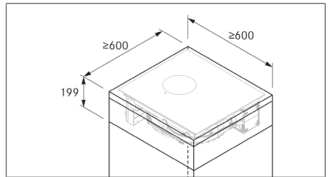
Abb. 11.4 Möbel-Mindestmaße S Pure
