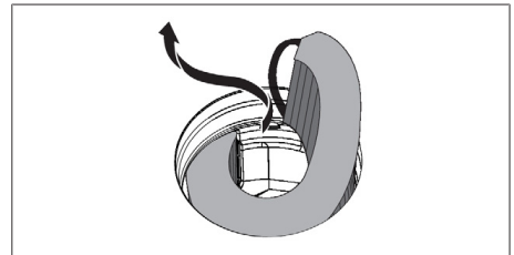
Abb. 9.6 Geruchsfilter aus der Einströmöffnung entnehmen
