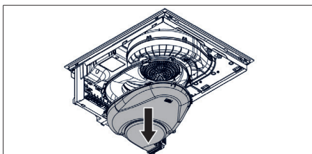
Abb. 11.28 Saugraum-Unterteil demontieren
