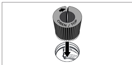
Abb. 9.8 Geruchsfilter in Abzugsöffnung einsetzen
