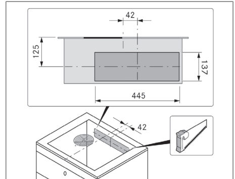
Abb. 11.15 Rückwand-Ausschnitt
