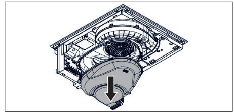
Fig. 11.28 Desmontaje de la parte inferior del espacio de aspiración
