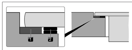
Fig. 11.24 Placas de compensación de altura
