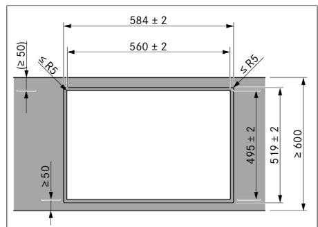
Fig. 11.9 Medidas del recorte para montaje enrasado
