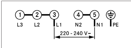
Fig. 11.31 Esquema de conexiones conexión monofásica
