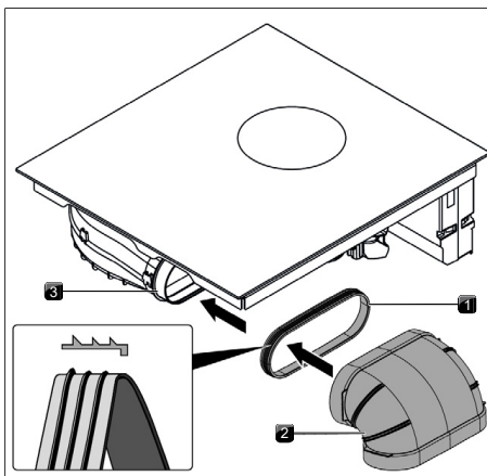
Fig. 11.25 Conexión al sistema de conductos
