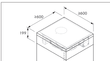
Fig. 11.4 Medidas mínimas de los muebles S Pure
