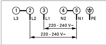
Fig. 11.30 Esquema de conexiones, conexión bifásica
