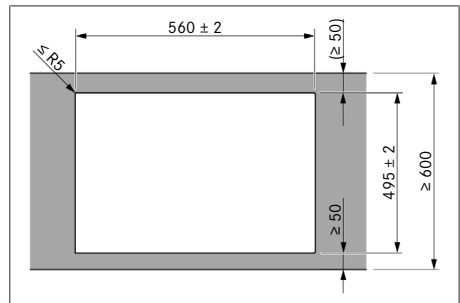
Fig. 11.7 Medidas del recorte para montaje superpuesto
