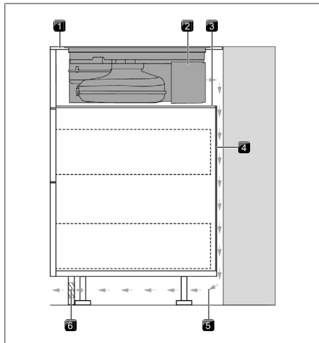
Fig. 11.14 Variante de montaje con base intermedia
