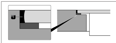
Fig. 11.39 Silicona de sellado para montaje enrasado
