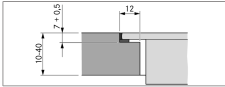
Fig. 11.10 Medida del rebaje para un montaje enrasado
