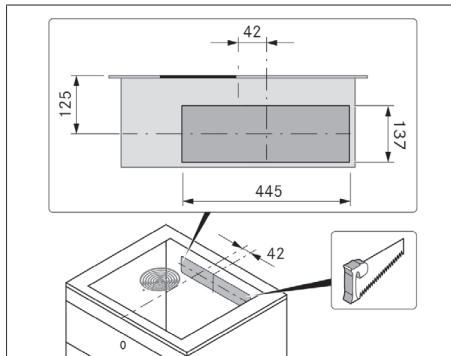
Fig. 11.15 Recorte del panel trasero
