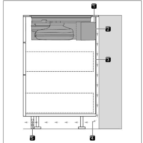
Fig. 11.13 Variante de montaje con panel trasero continuo
