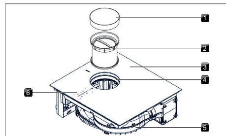
Fig. 4.1 Placa de cocción
