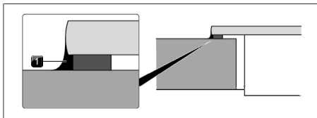
Fig. 11.38 Silicona de sellado para montaje superpuesto
