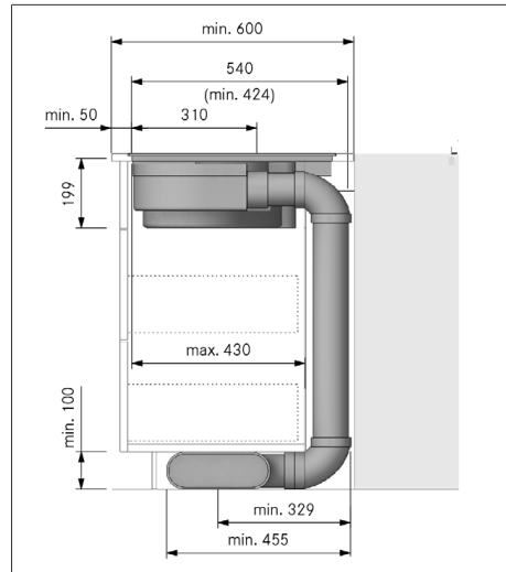
Fig. 11.11 Medidas de montaje para extracción al exterior, profundidad de la encimera 600 mm
