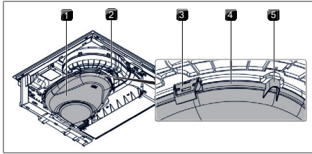
Fig. 9.3 Carcasa de conducción del aire
