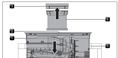
Fig. 11.21 Colocación de la placa de cocción
