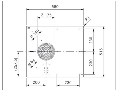
Fig. 3.1 Vista superior PURSA2/R
