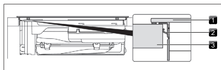
Fig. 11.22 Fijación de la placa de cocción en posición centrada
