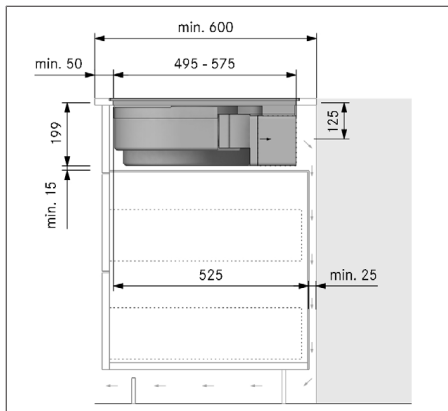
Fig. 11.18 Medidas de montaje para la variante de recirculación B, profundidad de la encimera 600 mm
