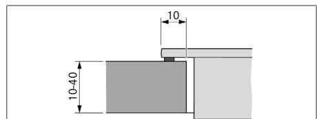
Fig. 11.8 Medida del apoyo para montaje superpuesto
