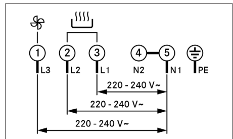
Fig. 11.29 Esquema de conexiones, conexión trifásica
