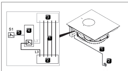
Fig. 11.33 Esquema de conexiones con contactos de conmutación externos
