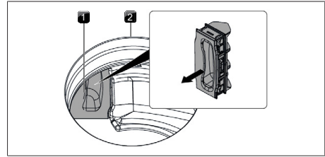
Fig. 9.4 Retirar la trampilla para el cambio del filtro
