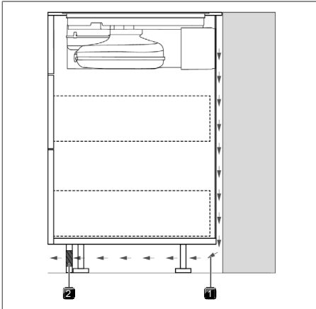
Fig. 11.12 Abertura de flujo de retorno en la zona del zócalo
