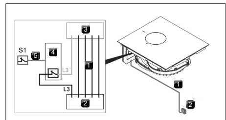
Sl. 11.33 Priključna shema z zunanjimi stikalnimi kontakti
