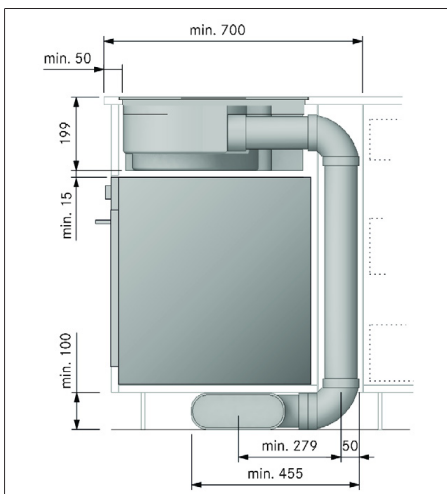
Sl. 11.6 PURSA2/R nad pečico z napeljavo kanala v območje podstavka
