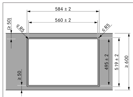
Sl. 11.9 Dimenzije izreza za montažo v isti ravnini s površino
