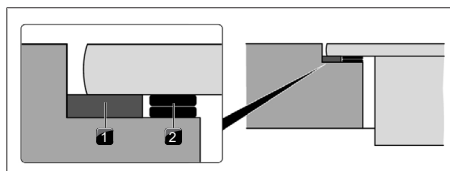
Sl. 11.24 Plošče za izravnavo višine
