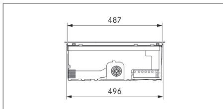
Sl. 3.6 Pogled od strani na PURSU2/R
