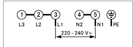
Sl. 11.31 Priključna shema enofaznega priključka
