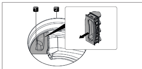
Sl. 9.4 Odstranitev lopute za zamenjavo filtra
