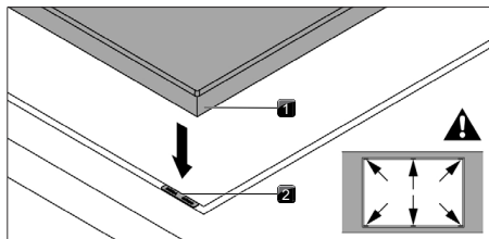
Sl. 11.23 Namestitev plošč za izravnavo višine
