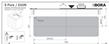
Sl. 11.16 Šablona za izrez hrbtišča
