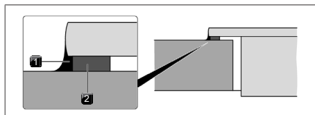
Sl. 11.19 Trak za tesnjenje pri nasadni montaži
