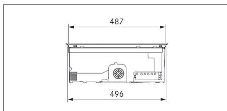
Sl. 3.3 Pogled od strani na PURSA2/R
