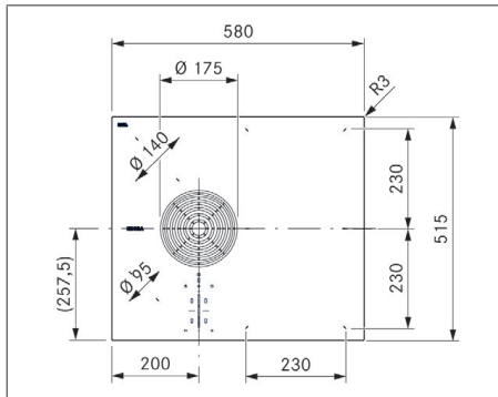
Sl. 3.4 Pogled od zgoraj na PURSU2/R
