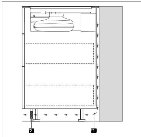
Sl. 11.12 Odprtina za povratni tok v območju vtiča
