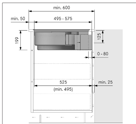
Sl. 11.17 Dimenzije vgradnje pri obtočnem zraku, različica montaže A
