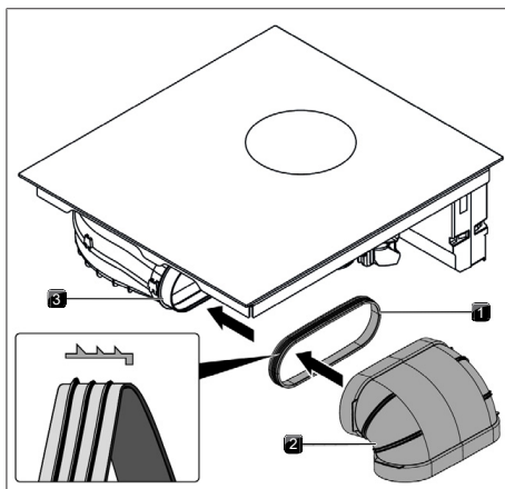
Sl. 11.25 Priključitev na sistem kanala
