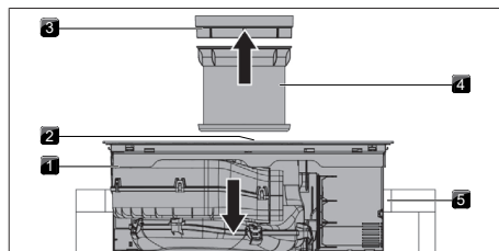
Sl. 11.21 Vstavljanje kuhalne plošče
