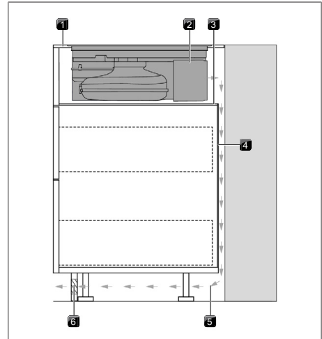
Sl. 11.14 Različica montaže z vmesnim dnom
