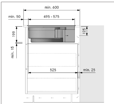
Sl. 11.18 Dimenzije vgradnje pri različici montaže B z obtočnim zrakom, globina delovne plošče 600 mm
