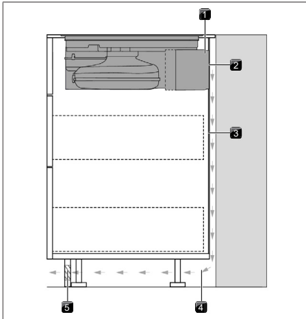
Sl. 11.13 Različica montaže s stalno zadnjo stranjo
