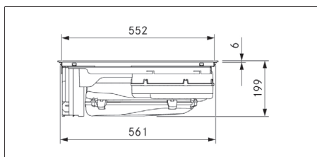
Sl. 3.2 Pogled od spredaj na PURSA2/R
