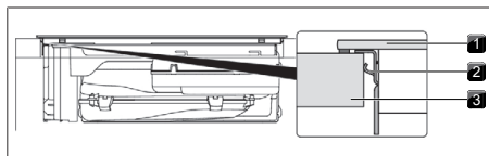
Sl. 11.22 Sredinsko pritrjevanje kuhalne plošče
