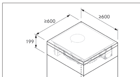
Sl. 11.4 Najmanjše dimenzije pohištva S Pure
