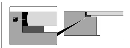
Sl. 11.39 Silikonska tesnilna masa pri montaži v isti ravnini s površino
