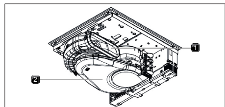
Sl. 4.2 Različica z odvodom zraka, pogled od zadaj
