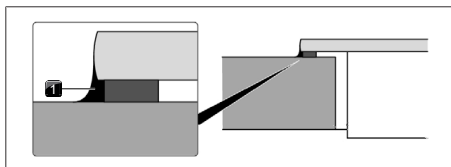
Sl. 11.38 Silikonska tesnilna masa pri nasadni montaži
