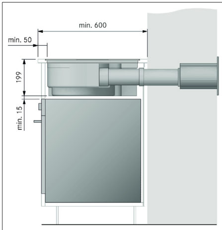
Sl. 11.5 PURSA2/R nad pečico z napeljavo za zrak naravnost nazaj v stensko škatlo
