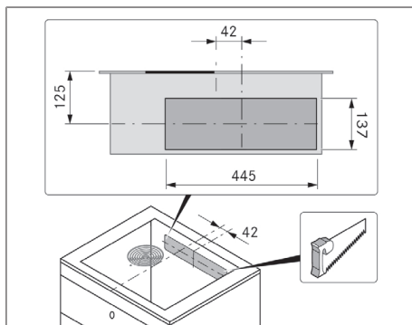
Sl. 11.15 Izrez hrbtišča
