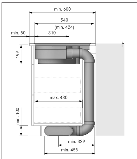
Sl. 11.11 Dimenzije vgradnje pri odvodu zraka, globina delovne plošče 600 mm
