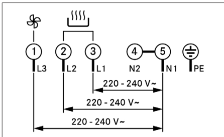
Sl. 11.29 Priključna shema trifaznega priključka
