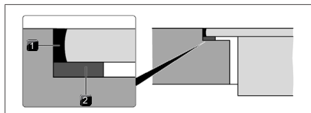
Sl. 11.20 Trak za tesnjenje pri montaži v isti ravnini s površino
