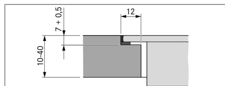
Sl. 11.10 Pregibna mera za montažo v isti ravnini s površino
