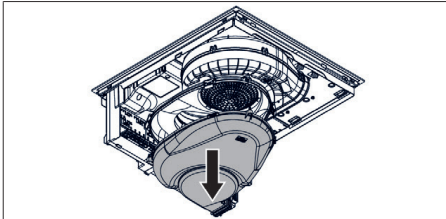
Sl. 11.28 Demontirajte spodnji del sesalne enote.
