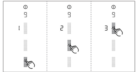
Sl. 8.10 Točka menija 9: Varnostni izklop
