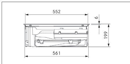
Sl. 3.5 Pogled od spredaj na PURSU2/R
