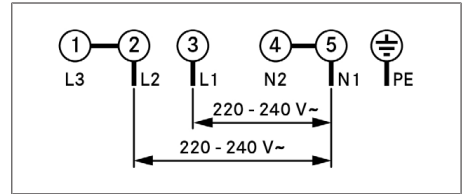
Sl. 11.30 Priključna shema dvofaznega priključka
