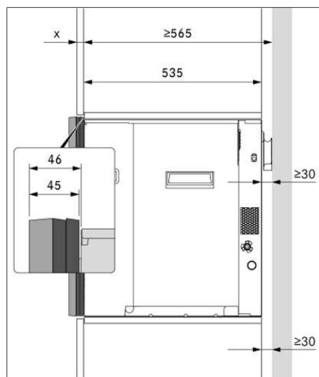
obr. 9.5 Montážní rozměry se 2 distančními rámy
