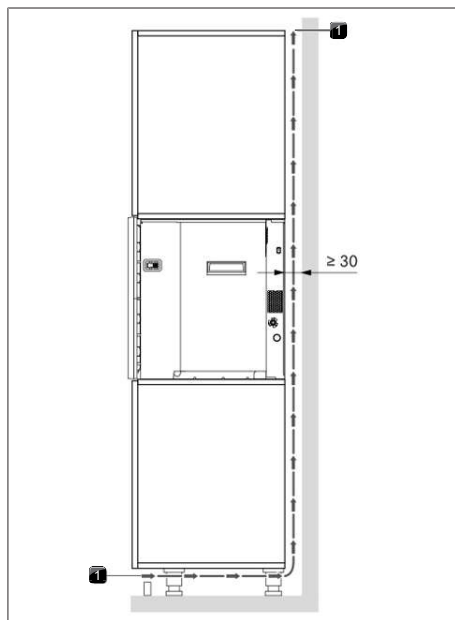
obr. 9.18 Větrání
