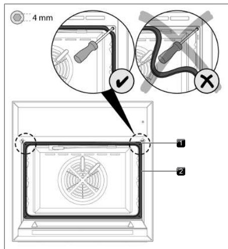
obr. 9.17 Připevnění spotřebiče
