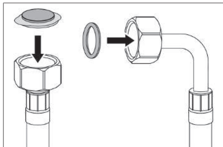
obr. 9.14 Hadice pro přívod vody s těsněním a sítkem k zachycování nečistot
