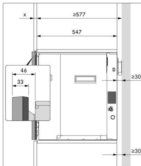
obr. 9.4 Montážní rozměry s 1 distančním rámem
