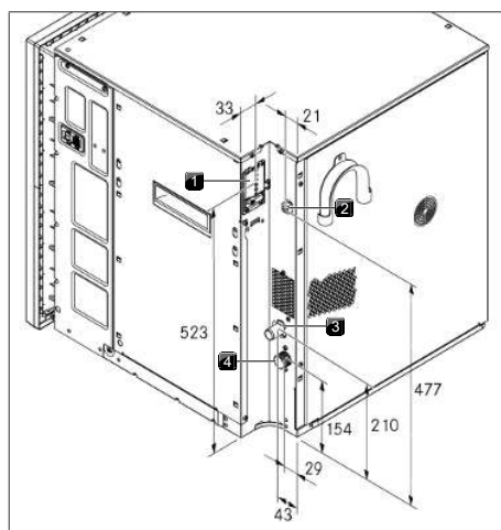
obr. 9.11 Přípojky zařízení
