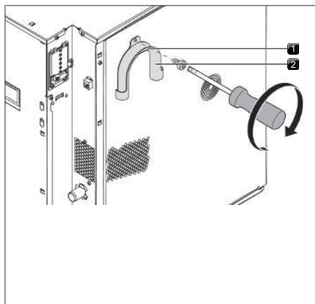
obr. 9.10 Haltebogen montieren
