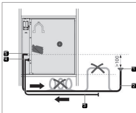
obr. 9.12 Odvod vody
