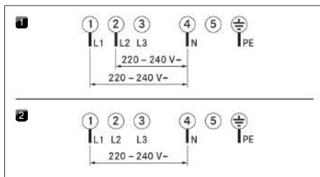
obr. 9.15 Schémata zapojení
