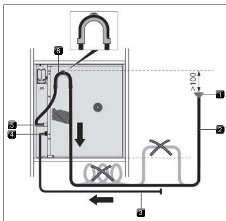
obr. 9.13 Odvod vody přes přídržné kolínko
