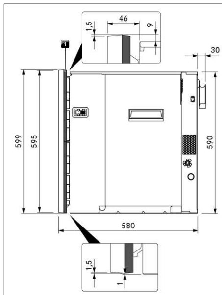
obr. 9.2 Rozměry
