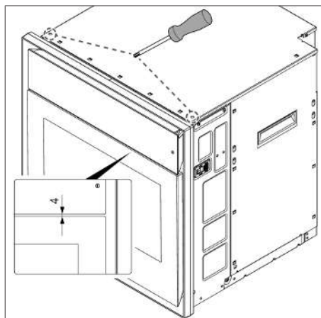
obr. 9.16 Nastavení vzdálenosti ovládací jednotky a dvířek
