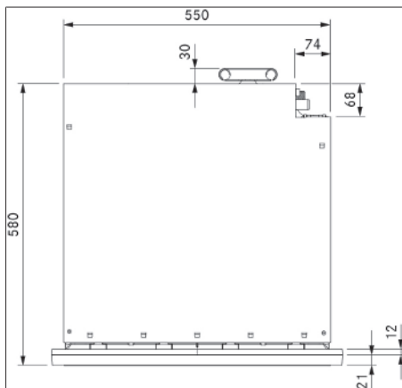
Kuva 3.2 XBO, kuva ylhäältä
