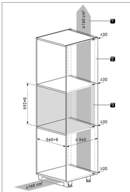
Kuva 9.1 Kalustekaappi
