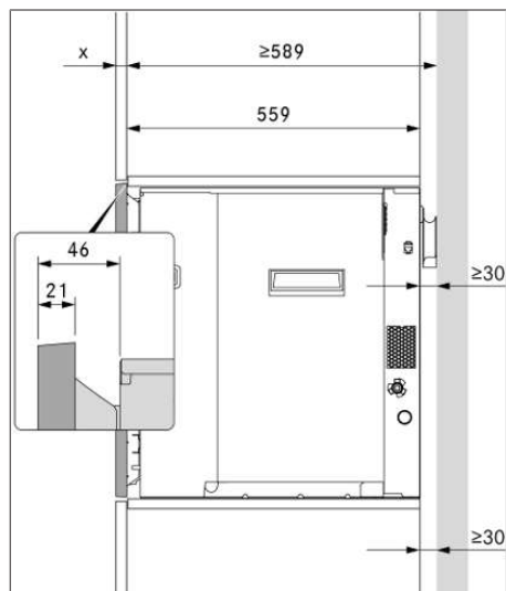
Kuva 9.3 Asennusmitat ilman kehysvälikettä
