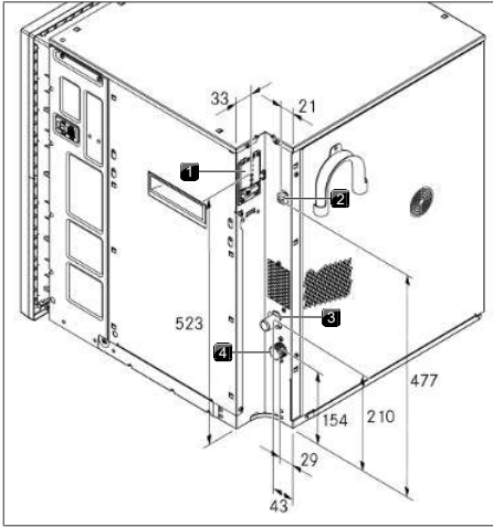
Kuva 9.11 Laitteen liitännät
