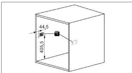
Kuva 9.9 Asennusaukko ja kalusteen kiinnityslevyt
