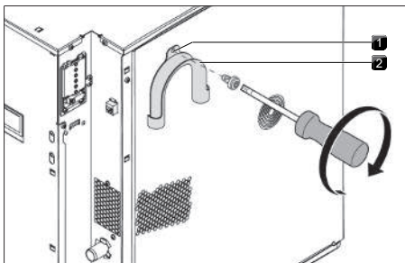
Kuva 9.10 Kannakekaaren asentaminen
