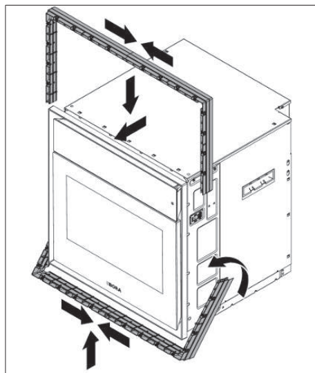
Kuva 9.8 2 kehysvälikkeen asennus
