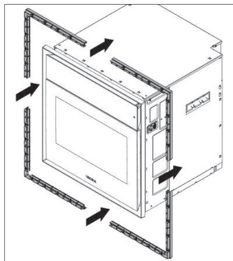
Kuva 9.6 Kehysvälikkeen irrottaminen
