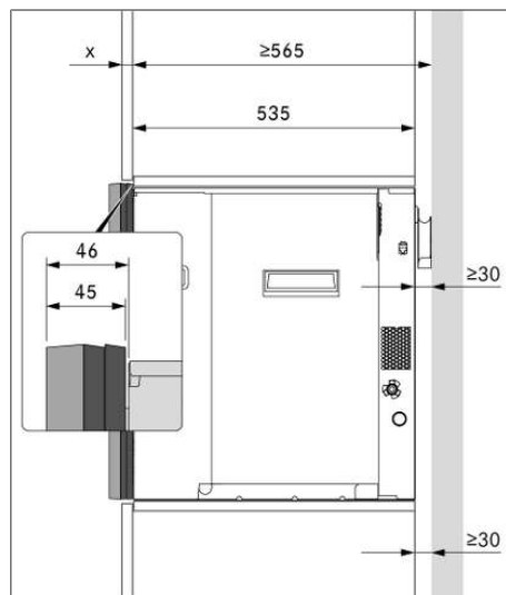
Kuva 9.5 Asennusmitat, 2 kehysvälikettä
