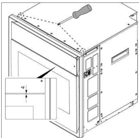
Kuva 9.16 Käyttöyksikön ja luukun välisen etäisyyden säätö
