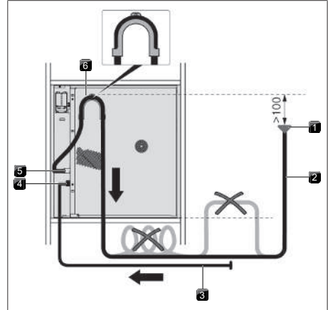
Kuva 9.13 Vedenpoisto kannakekaaren kautta
