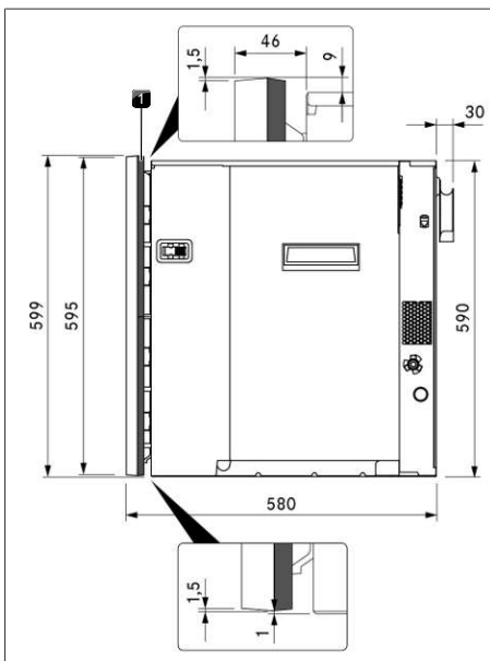
Kuva 9.2 Laitemitat
