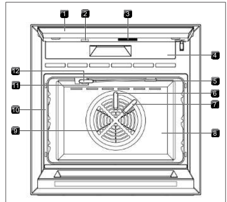
Kuva 4.1 Rakenne, osa 1
