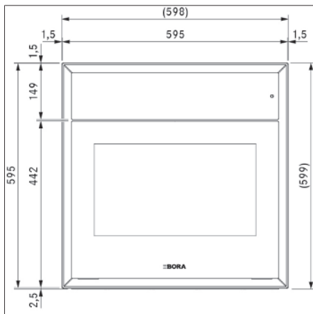
Kuva 3.1 XBO, kuva edestä
