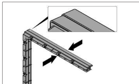
Kuva 9.7 2 kehysvälikeosaa
