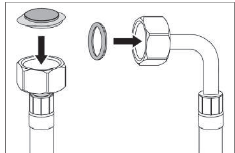
Kuva 9.14 Veden tuloletku, likasuodatin ja tiiviste
