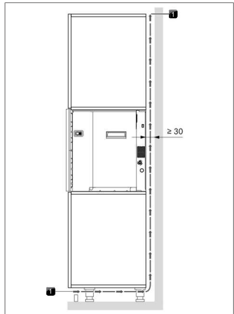
Kuva 9.18 Tuuletus
