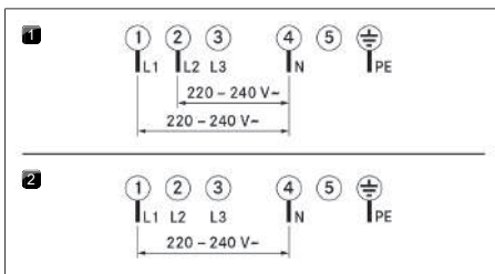
Kuva 9.15 Liitäntäkaaviot
