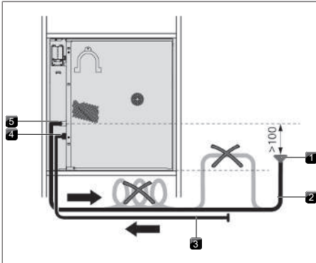
Kuva 9.12 Vedenpoisto
