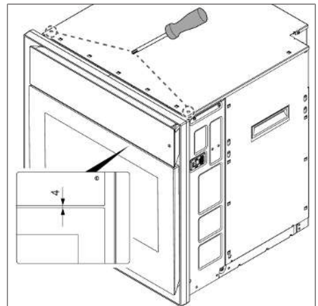
Fig. 9.16 Impostazione distanza unità di comando e porta
