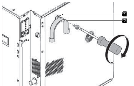
Fig. 9.10 Montaggio del raccordo
