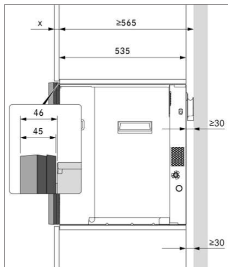
Fig. 9.5 Dimensioni di montaggio 2 distanziatori cornice
