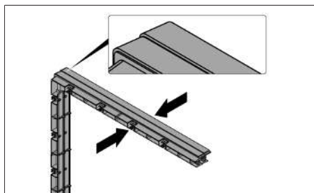
Fig. 9.7 2 elementi distanziatori cornice
