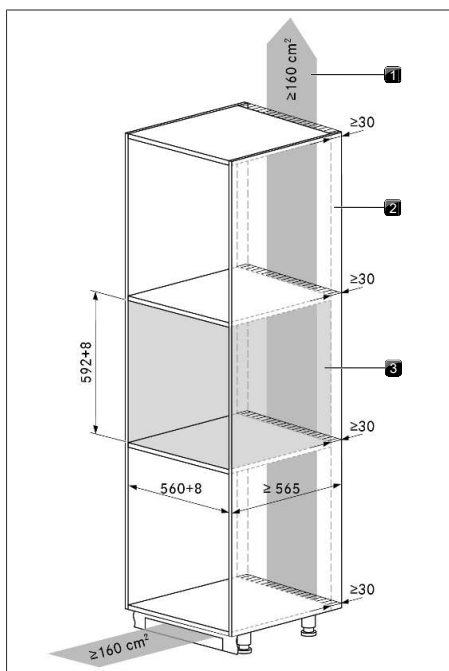
Fig. 9.1 Mobile da incasso
