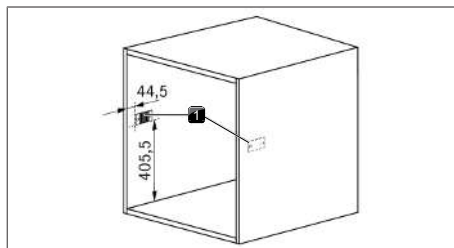
Fig. 9.9 Nicchia di montaggio con piastre a scatto del corpo
