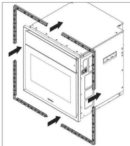
Fig. 9.6 Smontare il distanziatore cornice
