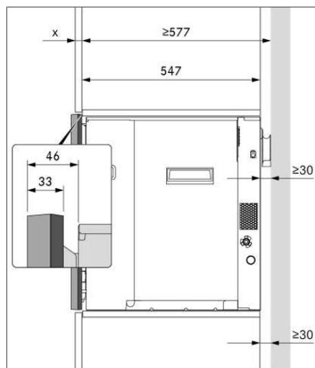
Fig. 9.4 Dimensioni di montaggio 1 distanziatori cornice
