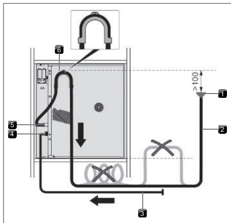
Fig. 9.13 Scarico dell'acqua sopra raccordo
