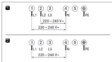
Fig. 9.15 Schemi di collegamento
