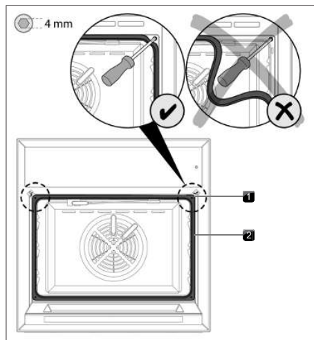
Fig. 9.17 Fissare l'apparecchio
