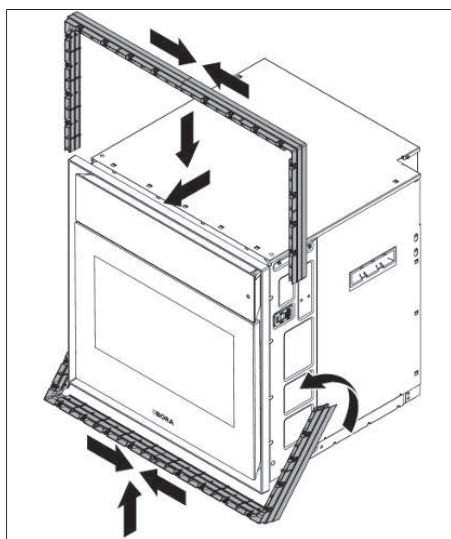
Fig. 9.8 Montare 2 distanziatori cornice
