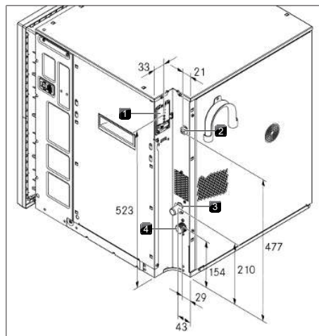
Fig. 9.11 Collegamento all'apparecchio
