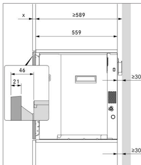
Fig. 9.3 Dimensioni di montaggio senza distanziatore cornice
