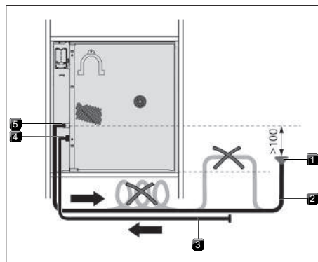
Fig. 9.12 Scarico dell'acqua
