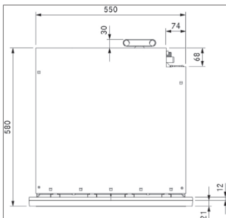
Fig. 3.2 Vista dall'alto XBO
