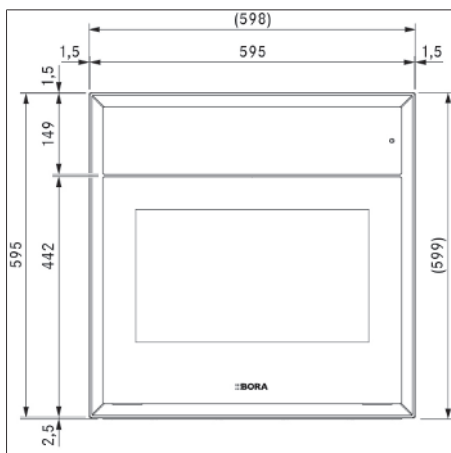
Fig. 3.1 Vista frontale XBO
