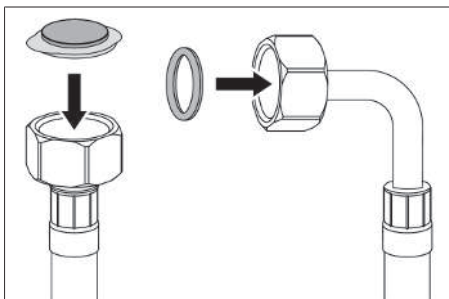
Fig. 9.14 Tubo di alimentazione dell'acqua con setaccio e guarnizione
