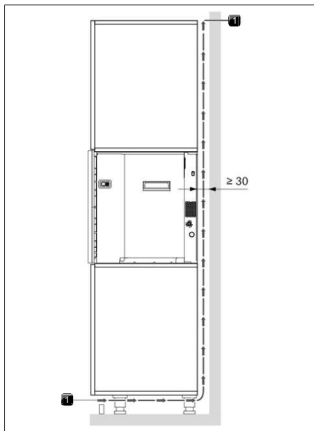
Fig. 9.18 Areazione
