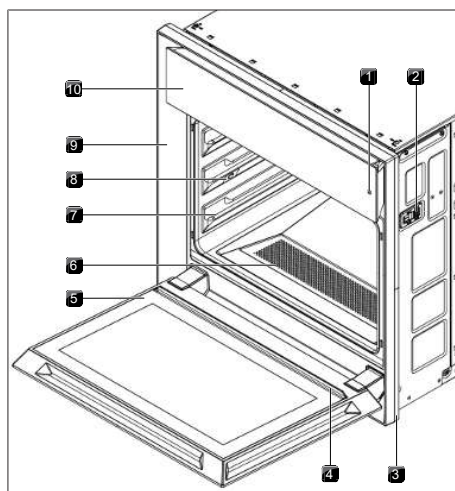
Fig. 4.2 Struttura parte 2
