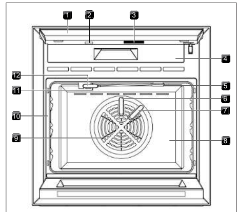
Fig. 4.1 Struttura parte 1
