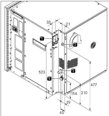
Afb. 9.11 Apparaataansluitingen
