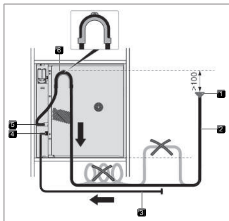
Afb. 9.13 Waterafvoer boven montagebocht
