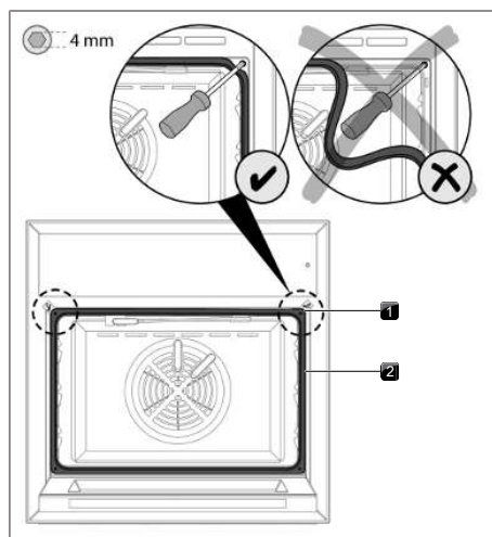
Afb. 9.17 Apparaat bevestigen
