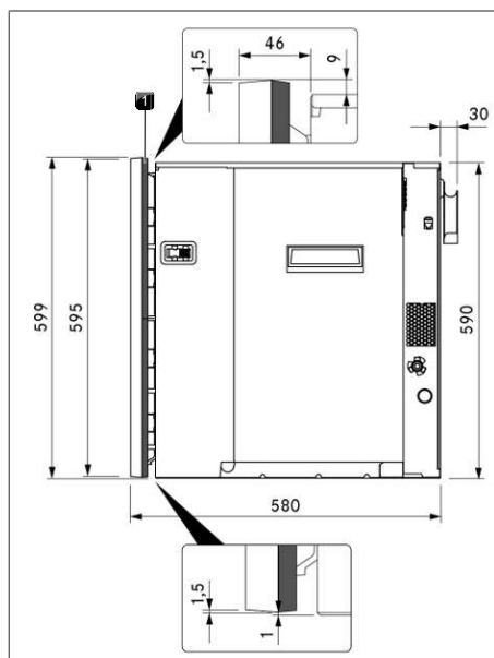
Afb. 9.2 Apparaatafmetingen
