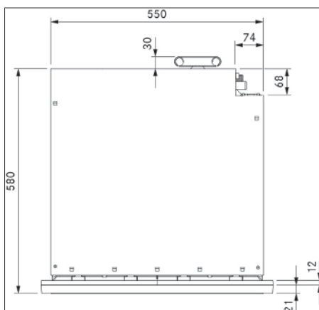
Afb. 3.2 Bovenaanzicht XBO
