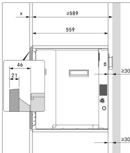
Afb. 9.3 Montageafmetingen zonder frame afstandhouder
