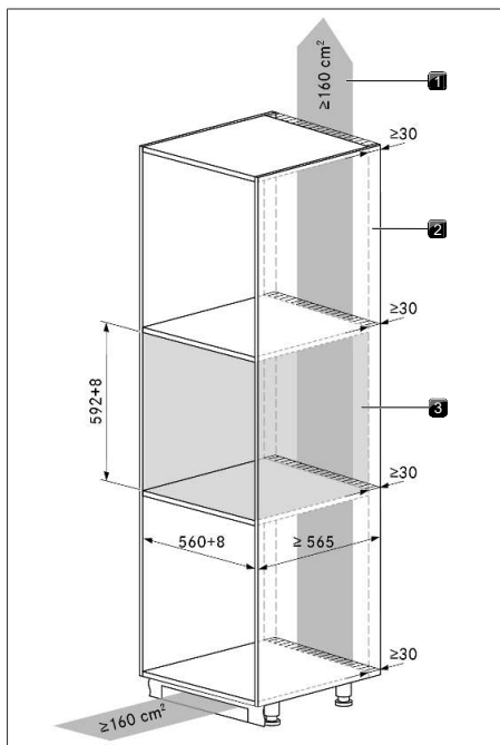
Afb. 9.1 Inbouwkast
