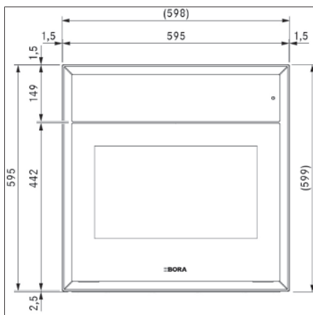
Afb. 3.1 Vooraanzicht XBO
