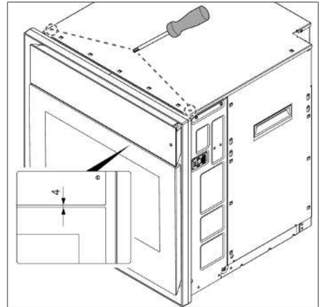
Afb. 9.16 Instellen van de afstand tussen de bedieningseenheid en de deur
