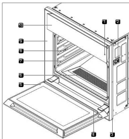
Afb. 4.2 Opbouw deel 2
