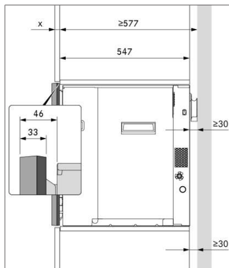
Afb. 9.4 Montageafmetingen 1 frame afstandhouders
