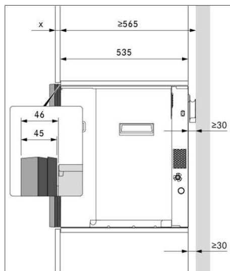
Afb. 9.5 Montageafmetingen 2 frame afstandhouders
