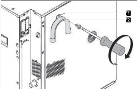
Afb. 9.10 Montagebocht plaatsen
