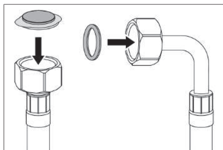
Afb. 9.14 Watertoevoerslang met vuilzeef en afdichting
