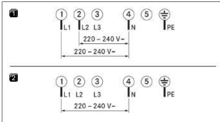
Afb. 9.15 Aansluitschema's
