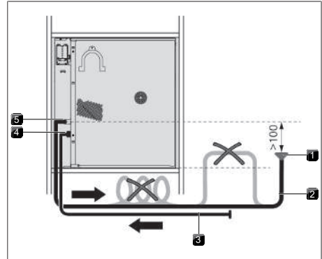
Afb. 9.12 Waterafvoer
