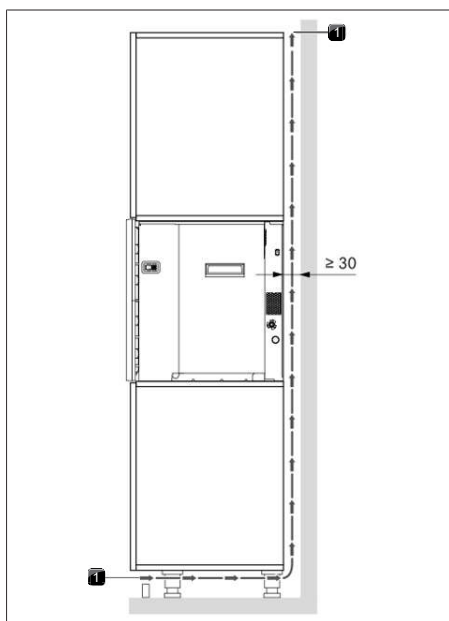
Afb. 9.18 Ventilatie
