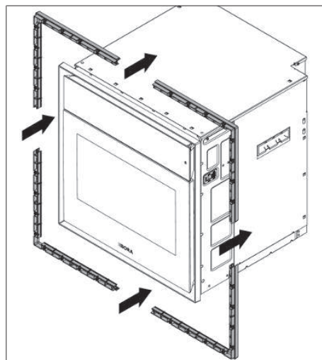
Fig. 9.6 Demontering av ramme-avstandsstykke
