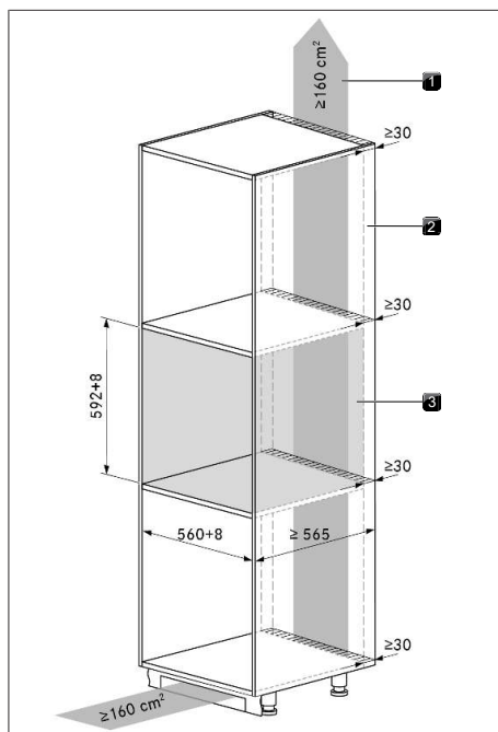
Fig. 9.1 Kjøkkenskap
