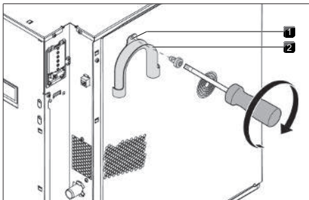
Fig. 9.10 Montere festevinkel
