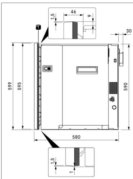
Fig. 9.2 Apparatdimensionen
