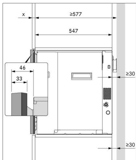
Fig. 9.4 Monteringsmål med 1 ramme-avstandsstykke
