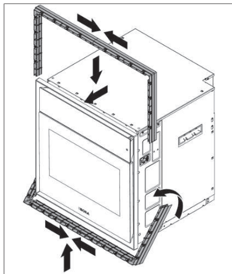
Fig. 9.8 Monter 2 ramme-avstandsstykker
