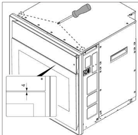
Fig. 9.16 Innstilling avstand betjeningsenhet og dør
