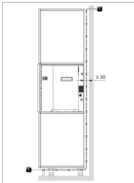
Fig. 9.18 Ventilasjon
