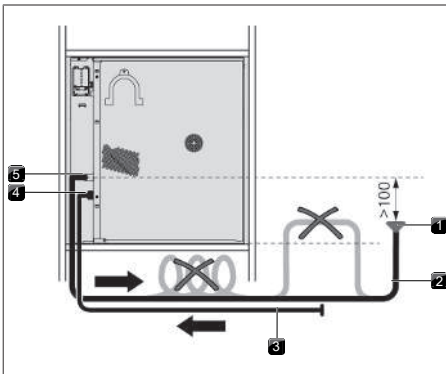
Fig. 9.12 Vannavløp
