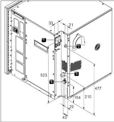
Fig. 9.11 Apparattilkoblinger
