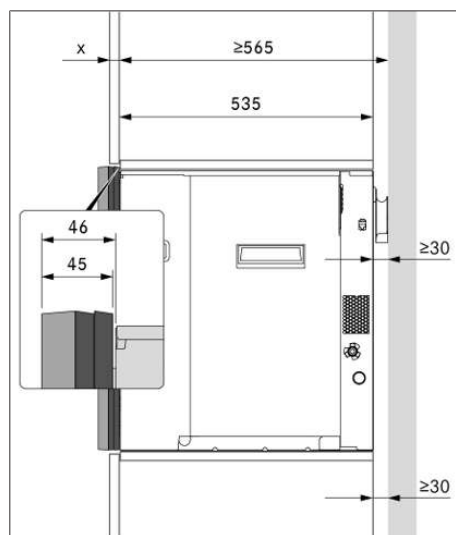
Fig. 9.5 Monteringsmål med 2 ramme-avstandsstykker
