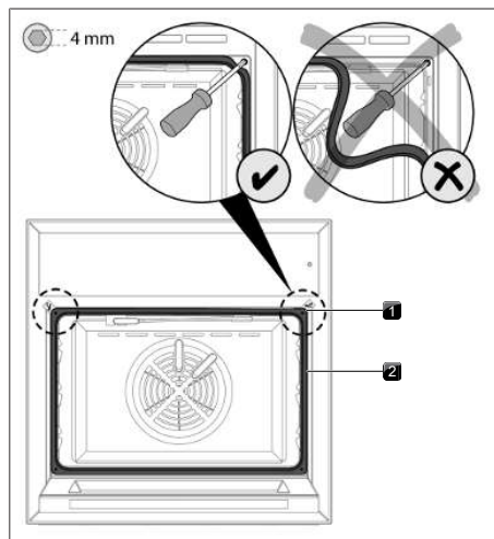
Fig. 9.17 Feste apparatet
