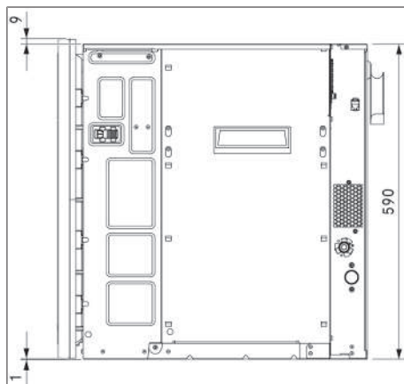
Fig. 3.3 Visning fra siden XBO
