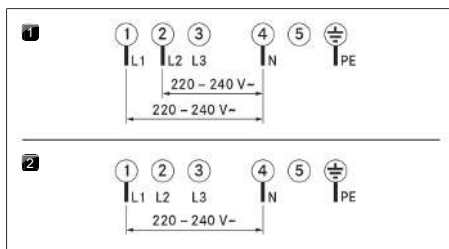
Fig. 9.15 Koblingsskjemaer
