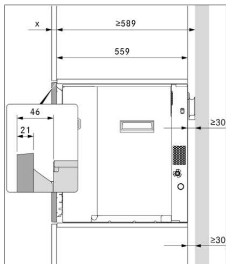
Fig. 9.3 Monteringsmål uten ramme-avstandsstykke
