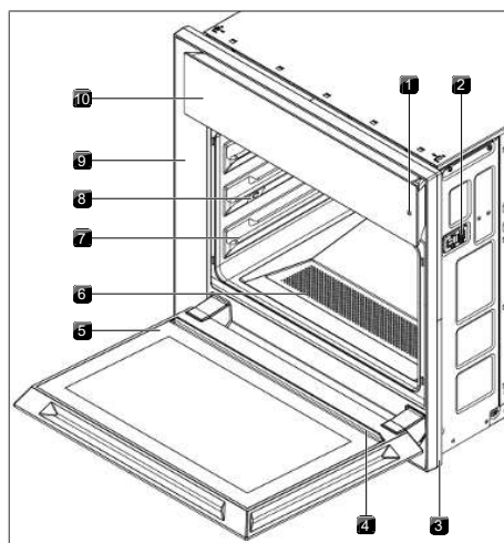
Fig. 4.2 Oppbygning del 2
