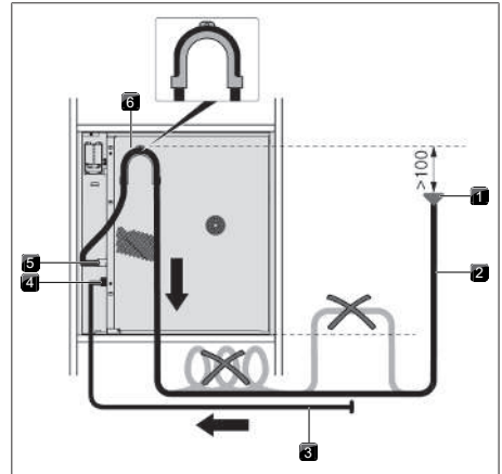
Fig. 9.13 Vannavløp over festevinkel
