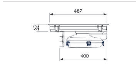
Fig. 3.3 PUXA2/R - enhedens mål set fra siden
