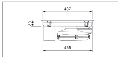
Fig. 3.6 PUXU2/R - enhedens mål set fra siden
