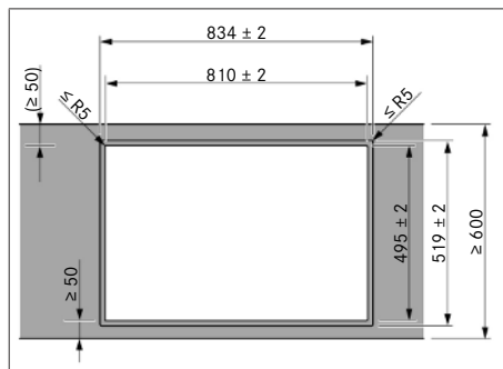
Fig. 11.5 Udskæringsmål til planlimet montage
