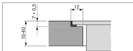
Fig. 11.6 Falsmål til planlimet montage
