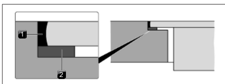
Fig. 11.18 Forseglingsstape til planlimet montering
