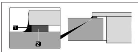
Fig. 11.17 Forseglingsstape ved overflademontering
