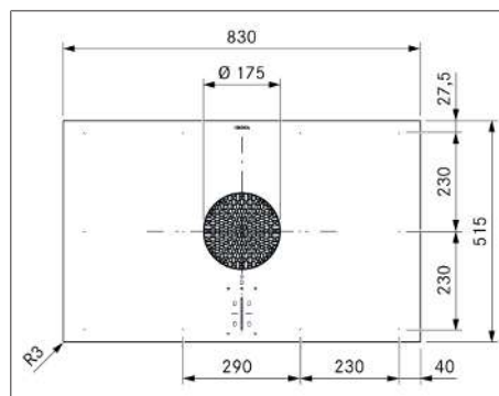
Fig. 3.1 PUXA2/R - enhedens mål set fra oven
