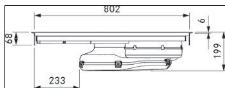
Fig. 3.2 PUXA2/R - enhedens mål set forfra
