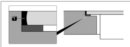
Fig. 11.36 Silikoneforseglingsmasse ved planlimet montage
