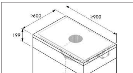
Fig. 11.4 Møbel mindstemål X Pure
