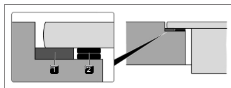
Fig. 11.22 Højdeudligningsplader
