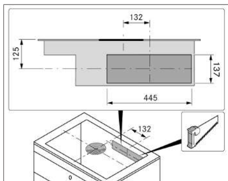
Fig. 11.11 Udsæring i bagvæggen
