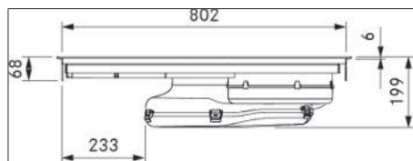
Fig. 3.5 PUXU2/R - enhedens mål set forfra
