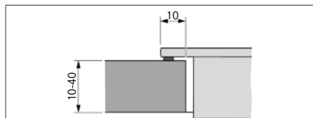
Fig. 11.8 Monteringsmål til overflademontage
