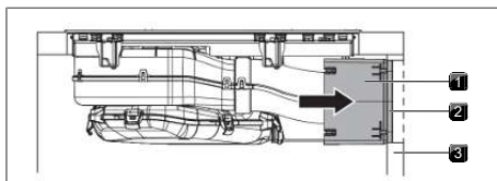
Fig. 11.25 Tilslutning til bagvæggen
