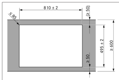
Fig. 11.7 Udskæringsmål til overflademontage
