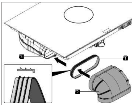
Fig. 11.24 Tilslutning til kanalsystem
