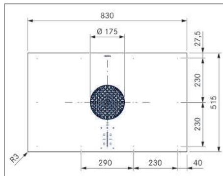
Fig. 3.4 PUXU2/R - enhedens mål set fra oven
