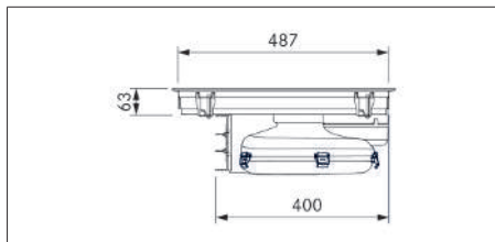
Fig. 3.3 Dimensions PUXA2/R - Vue latérale
