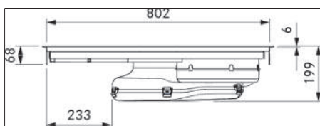
Fig. 3.2 Dimensions PUXA2/R - Vue de devant
