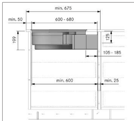
Fig. 11.14 Cotes de montage pour le recyclage d'air, variante A, profondeur du plan de travail à partir de 675 mm
