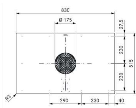
Fig. 3.1 Dimensions PUXA2/R - Vue de dessus
