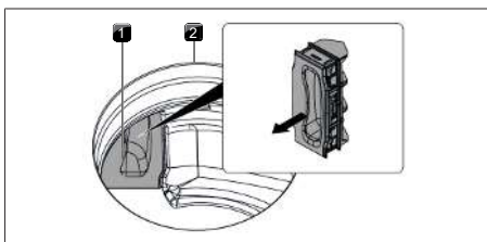
Fig. 9.4 Retrait du clapet de changement de filtre
