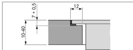
Fig. 11.6 Dimension de rainure pour montage affleurant
