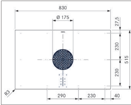
Fig. 3.4 Dimensions PUXU2/R - Vue de dessus
