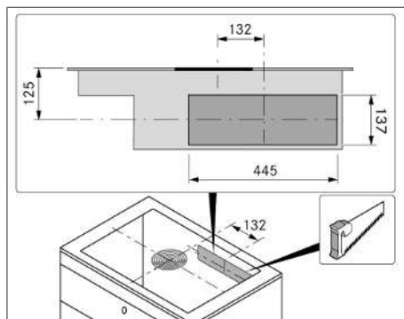
Fig. 11.11 Découpe dans la paroi arrière
