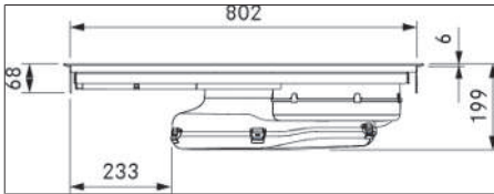
Fig. 3.5 Dimensions PUXU2/R - Vue de devant
