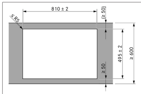
Fig. 11.7 Dimensions de découpe pour montage en saillie
