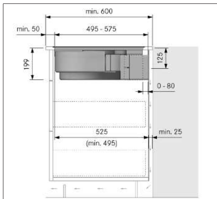
Fig. 11.13 Cotes de montage pour le recyclage d'air, variante A
