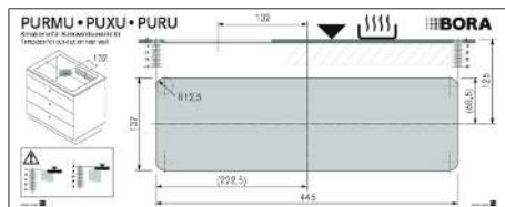
Fig. 11.12 Gabarit de découpe dans la paroi arrière
