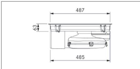
Fig. 3.6 Dimensions PUXU2/R - Vue latérale
