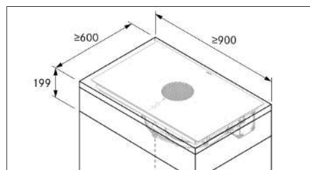
Fig. 11.4 Dimensions minimales du meuble pour X Pure
