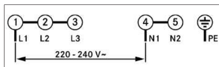
Fig. 11.28 Schema di collegamento monofase
