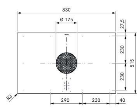
Fig. 3.1 PUXA2/R dimensioni apparecchio vista dall'alto
