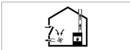
Fig. 11.2 Montaggio scarico aria – corretto
