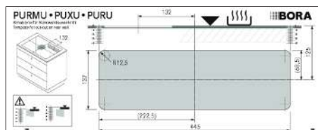
Fig. 11.12 Maschera per intaglio parete posteriore
