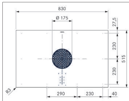
Fig. 3.4 PUXU2/R dimensioni apparecchio vista dall'alto
