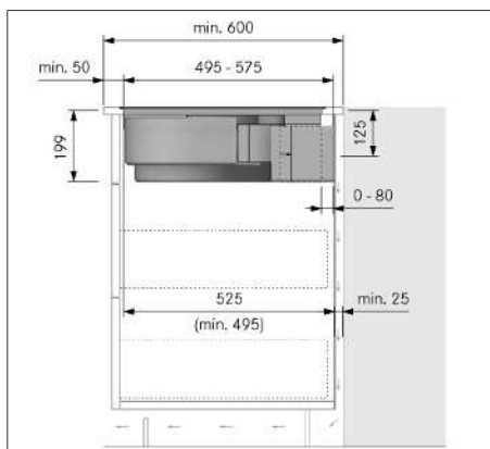
Fig. 11.13 Dimensioni di montaggio con sistema filtrante, variante di montaggio A
