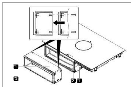
Fig. 11.15 Estensione della prolunga telescopica
