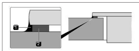
Fig. 11.17 Nastro a tenuta per montaggio in battuta
