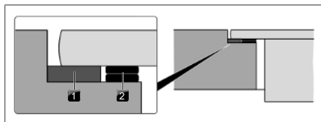
Fig. 11.22 Pannelli di compensazione altezza
