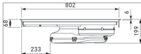
Fig. 3.2 PUXA2/R dimensioni apparecchio vista frontale
