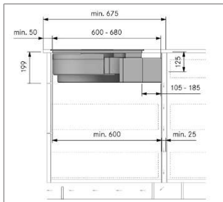
Fig. 11.14 Dimensioni di montaggio con sistema filtrante variante di montaggio A, profondità piano di lavoro da 675 mm
