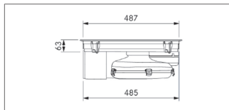
Fig. 3.6 PUXU2/R dimensioni apparecchio vista laterale
