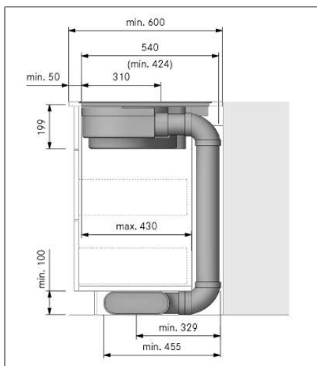
Fig. 11.9 Dimensioni di montaggio con sistema aspirante, profondità piano di lavoro 600 mm
