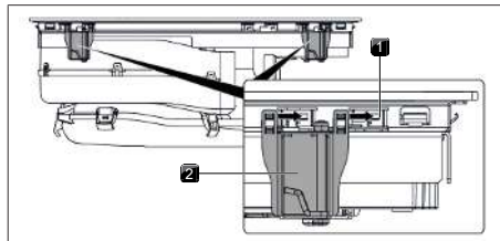
Fig. 11.19 Applicare i morsetti di montaggio
