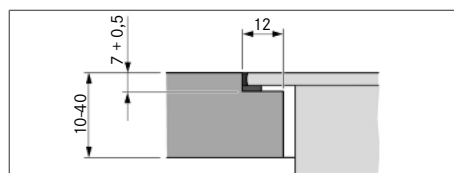
Fig. 11.6 Dimensioni dell'incassatura per montaggio a filo piano
