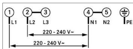
Fig. 11.29 Schema di collegamento bifase
