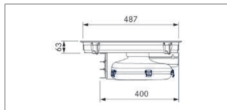
Fig. 3.3 PUXA2/R dimensioni apparecchio vista laterale
