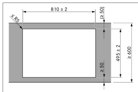
Fig. 11.7 Dimensioni intaglio per montaggio in battuta
