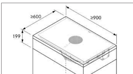
Fig. 11.4 Dimensioni minime mobili X Pure
