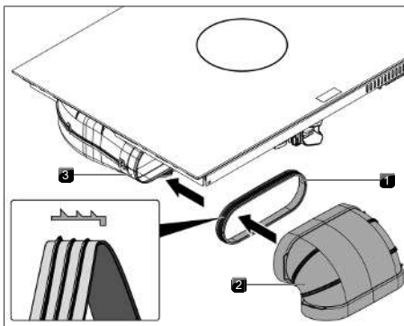
Fig. 11.24 Connessione al sistema di canali
