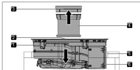
Fig. 11.20 Inserire il piano cottura nel centro
