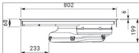
Fig. 3.5 PUXU2/R dimensioni apparecchio vista frontale
