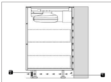
Fig. 11.10 Apertura di sfogo nell'area dello zoccolo
