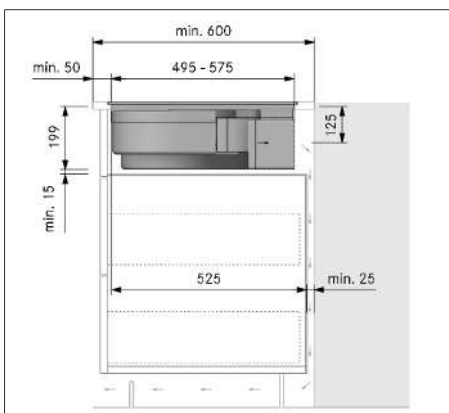
Fig. 11.16 Dimensioni di montaggio con sistema filtrante variante di montaggio B, profondità piano di lavoro 600 mm
