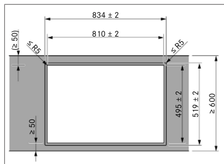
Fig. 11.5 Dimensioni intaglio per montaggio a filo
