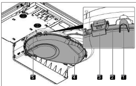
Fig. 9.3 Alloggiamento condotta aria
