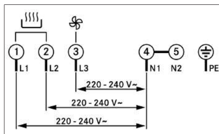
Fig. 11.27 Schema di collegamento trifase
