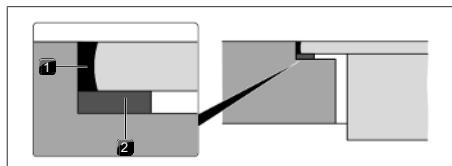
Fig. 11.18 Nastro a tenuta per montaggio a filo piano
