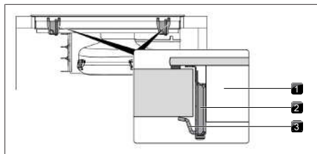
Fig. 11.23 Fissare il piano cottura nel centro
