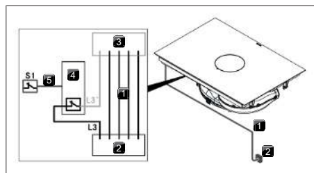
Fig. 11.26 Schema di collegamento con contatto di commutazione esterno
