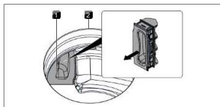
Fig. 9.4 Rimuovere la valvola di sostituzione del filtro
