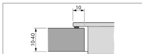
Fig. 11.8 Misura d'appoggio per montaggio in battuta
