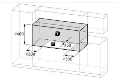
Fig. 11.3 Spazio libero necessario
