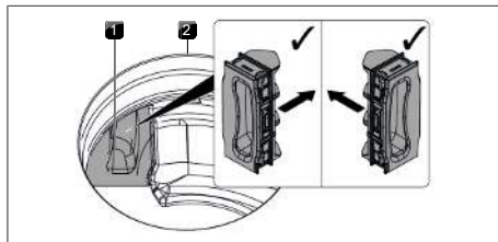
Fig. 9.10 Inserire la valvola di sostituzione del filtro
