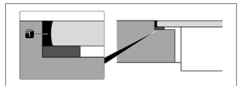
Fig. 11.36 Pasta sigillante al silicone per montaggio a filo piano
