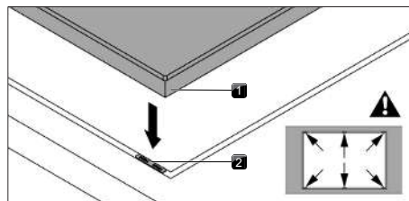
Fig. 11.21 Posizionamento dei pannelli di compensazione altezza
