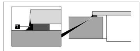
Fig. 11.35 Pasta sigillante al silicone per montaggio in battuta
