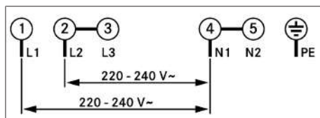
Afb. 11.29 Aansluitschema 2-faseaansluiting
