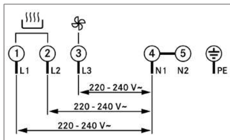
Afb. 11.27 Aansluitschema 3-faseaansluiting
