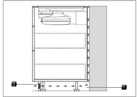
Afb. 11.10 Terugstroomopening in plintgedeelte
