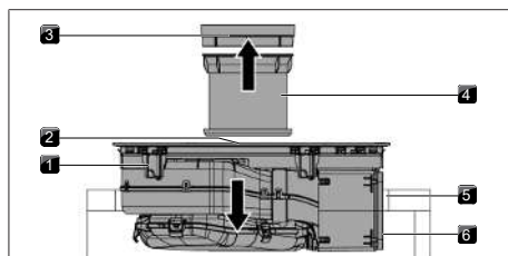
Afb. 11.20 Centrale plaatsing kookveld
