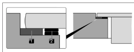
Afb. 11.22 Vulplaatjes
