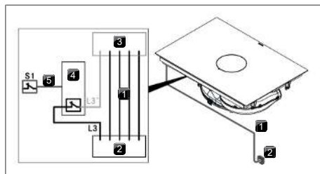
Afb. 11.26 Aansluitschema met extern schakelcontact
