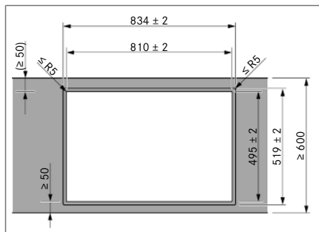
Afb. 11.5 Uitsparingsafmetingen in geval van vlakinbouw
