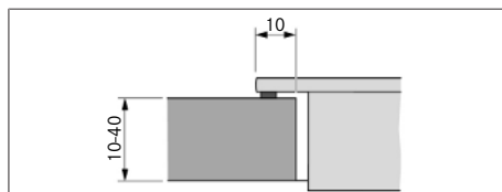
Afb. 11.8 Oplegmaat voor opbouwmontage
