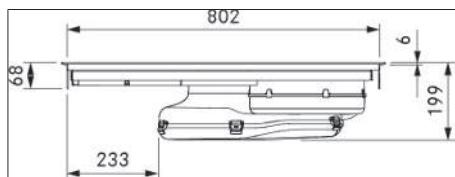
Afb. 3.5 PUXU2/R toestelafmetingen vooraanzicht
