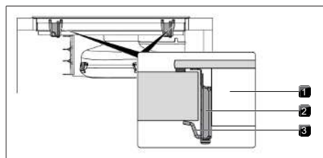
Afb. 11.23 Centrale bevestiging kookveld
