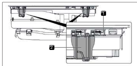
Afb. 11.19 Montageklemmen aanbrengen
