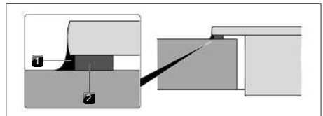
Afb. 11.17 Afdichtingsband bij opbouwmontage
