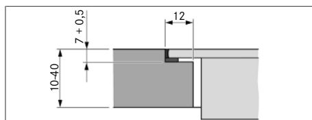
Afb. 11.6 Voegmaat voor vlakinbouw
