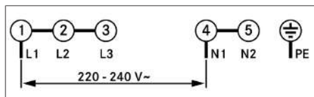
Afb. 11.28 Aansluitschema 1-faseaansluiting
