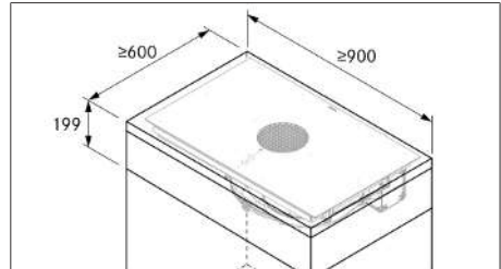
Afb. 11.4 Minimale meubelafmetingen X Pure
