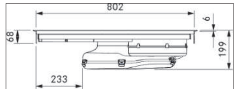
Afb. 3.2 PUXA2/R toestelafmetingen vooraanzicht
