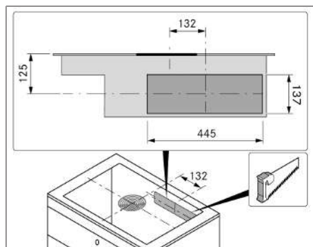
Afb. 11.11 Achterwanduitsparing
