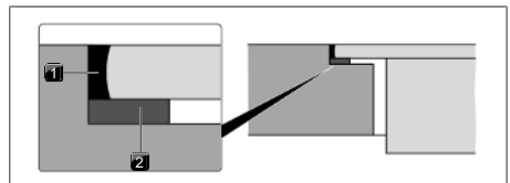
Afb. 11.18 Afdichtingsband bij vlaginbouw
