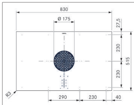
Afb. 3.4 PUXU2/R toestelafmetingen bovenaanzicht
