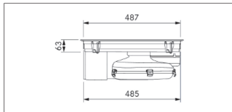
Afb. 3.6 PUXU2/R toestelafmetingen zijaanzicht
