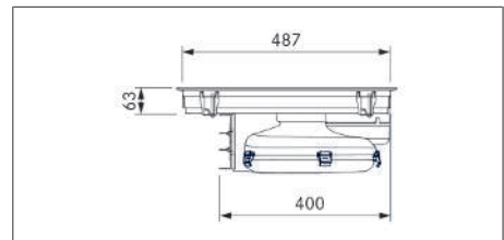
Afb. 3.3 PUXA2/R toestelafmetingen zijaanzicht
