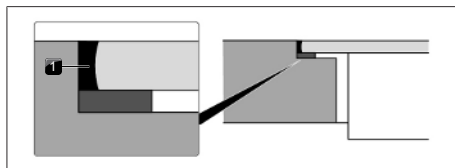
Afb. 11.36 Siliconenkit bij vlakbouw
