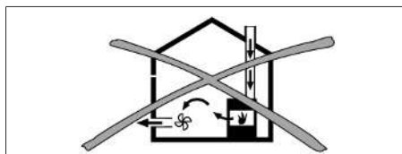
Afb. 11.1 Montage mit Luftabfuhr – niet toegestaan
