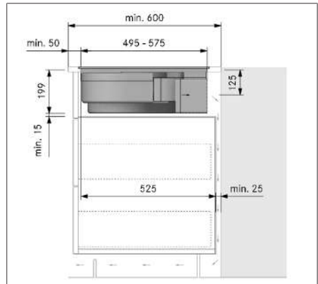
Afb. 11.16 Inbouwmaten bij recirculatie - montagevariant B, werkbladdiepte 600 mm
