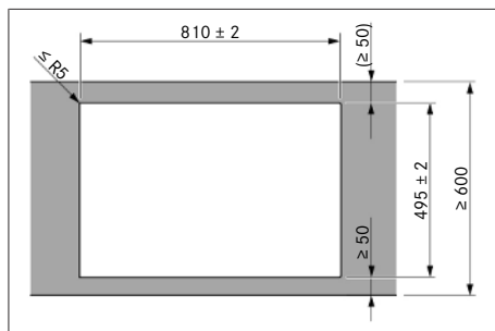
Afb. 11.7 Uitsparingsafmetingen in geval van opbouwmontage
