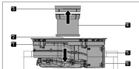
Fig. 11.20 Colocar a placa de cozinhar centrada
