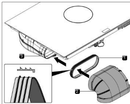
Fig. 11.24 Ligação ao sistema de condutas
