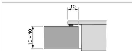
Fig. 11.8 Medida do apoio para montagem por sobreposição
