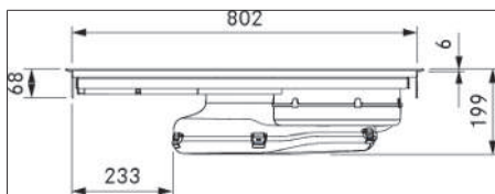
Fig. 3.2 PUXA2/R dimensões do aparelho vista frontal
