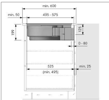
Fig. 11.13 Medidas de montagem para a recirculação de ar, variante de montagem A
