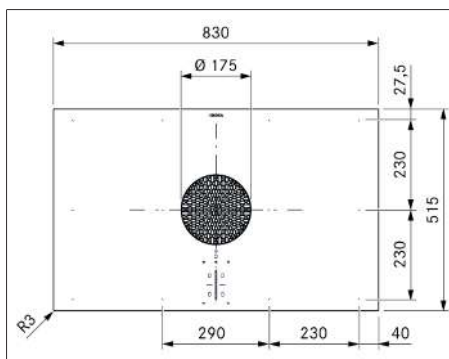
Fig. 3.1 PUXA2/R dimensões do aparelho vista de cima
