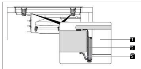
Fig. 11.23 Fixar a placa de cozinhar centrada
