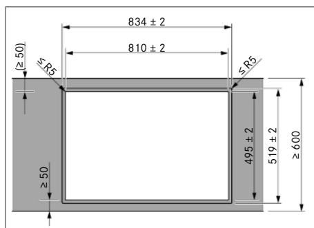
Fig. 11.5 Medidas de recorte para montagem à face
