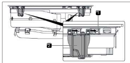
Fig. 11.19 Instalar grampos de montagem
