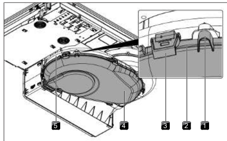
Fig. 9.3 Carcaça de condução do ar
