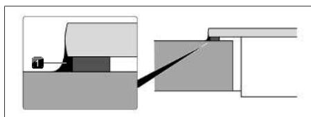
Fig. 11.35 Massa vedante de silicone na montagem por sobreposição
