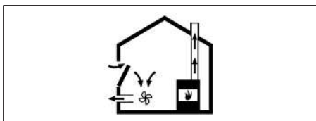
Fig. 11.2 Montagem do sistema de extração de ar – correta
