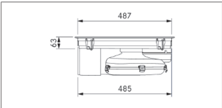
Fig. 3.6 PUXU2/R dimensões do aparelho vista lateral
