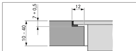
Fig. 11.6 Medida de recesso para montagem à face
