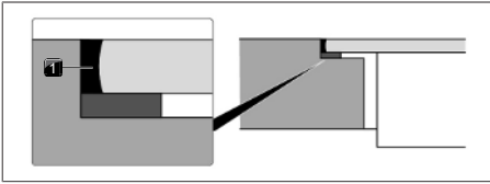
Fig. 11.36 Massa vedante de silicone na montagem à face
