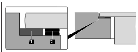
Fig. 11.22 Placas de compensação de altura
