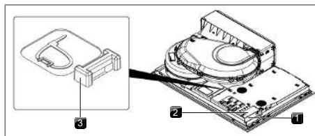
Fig. 11.30 Ligações elétricas da placa de cozinhar
