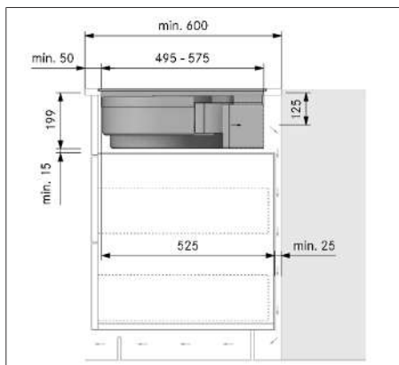
Fig. 11.16 Medidas de montagem para a circulação de ar, variante de montagem B, profundidade da bancada de 600 mm
