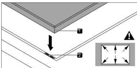
Fig. 11.21 Posicionamento e placas de compensação de altura
