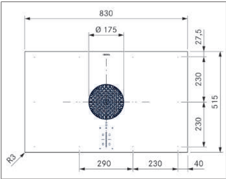
Fig. 3.4 PUXU2/R dimensões do aparelho vista de cima
