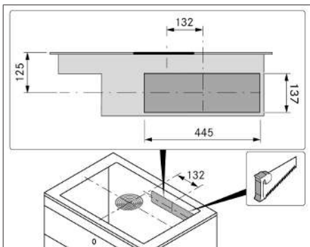
Fig. 11.11 Recorte do painel traseiro
