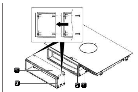
Fig. 11.15 Extensão da guia telescópica
