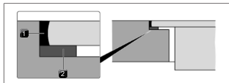
Fig. 11.18 Cinta vedante na montagem à face
