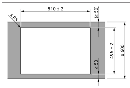
Fig. 11.7 Medidas de recorte para montagem por sobreposição
