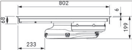
Fig. 3.5 PUXU2/R dimensões do aparelho vista frontal
