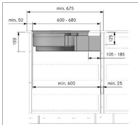
Fig. 11.14 Medidas de montagem para a recirculação de ar, variante de montagem A, profundidade da bancada a partir de 675 mm
