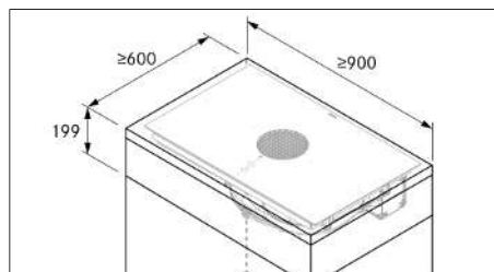
Fig. 11.4 Dimensões mínimas do móvel X Pure
