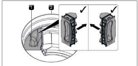
Fig. 9.10 Inserir a tampa de troca do filtro
