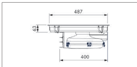
Fig. 3.3 PUXA2/R dimensões do aparelho vista lateral
