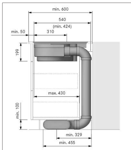
Fig. 11.9 Medidas de montagem para extração de ar, profundidade da bancada de 600 mm
