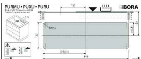
Fig. 11.12 Molde para o recorte do painel traseiro
