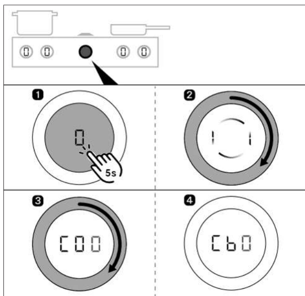
Fig. 6.5 Hente frem konfigurasjonsmenyen
