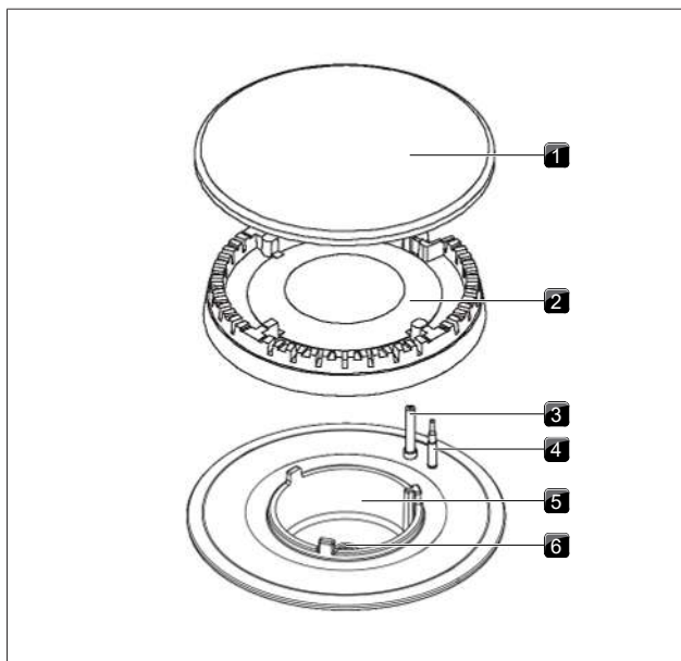
Fig. 7.7 Gassbrenner oppbygning
