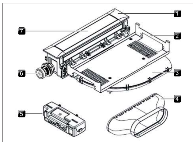
Fig. 3.5 Avtrekk PKA3/PKA3AB
