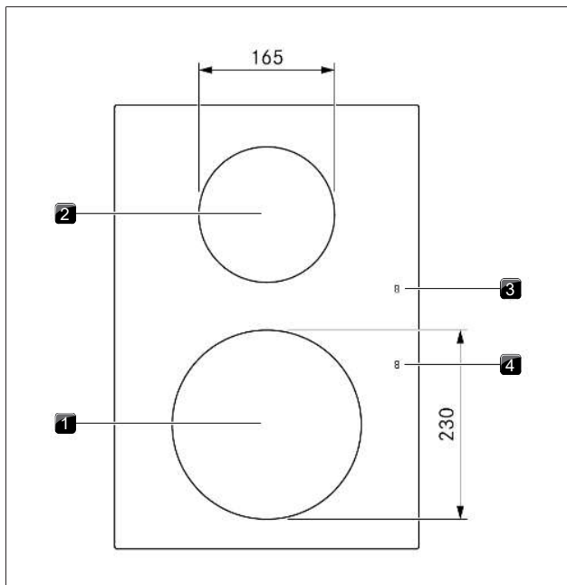
Fig. 3.9 Konstruksjon platetopp PKI3 og kokesonenes størrelse
