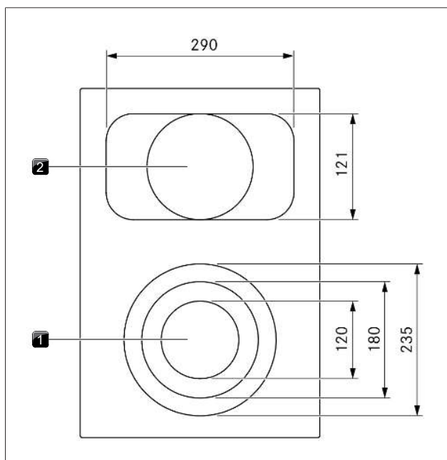
Fig. 3.12 Konstruksjon platetopp PKCB3 og kokesonenes størrelse
