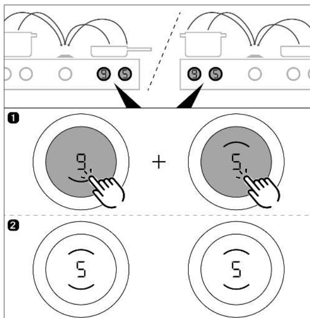
Fig. 5.26 Aktivere brofunksjon
