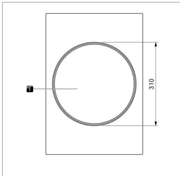
Fig. 3.10 Konstruksjon platetopp PKIW3 og kokesonenes størrelse
