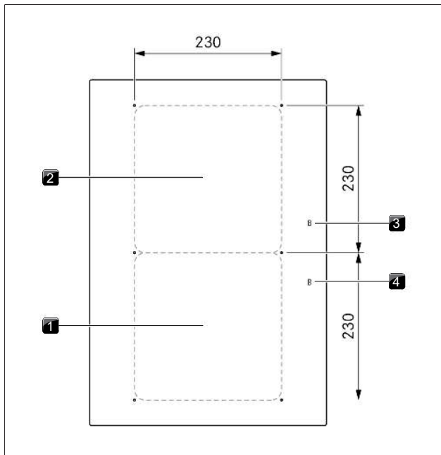
Fig. 3.8 Konstruksjon platetopp PKFI3 / PKFI3R og kokesonenes størrelse
