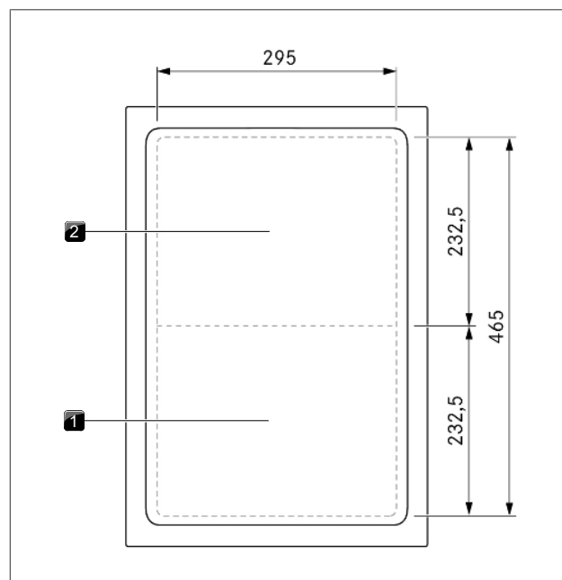
Fig. 3.14 Konstruksjon Tepan-grill i rustfritt stål PKT3 og kokesonenes størrelse
