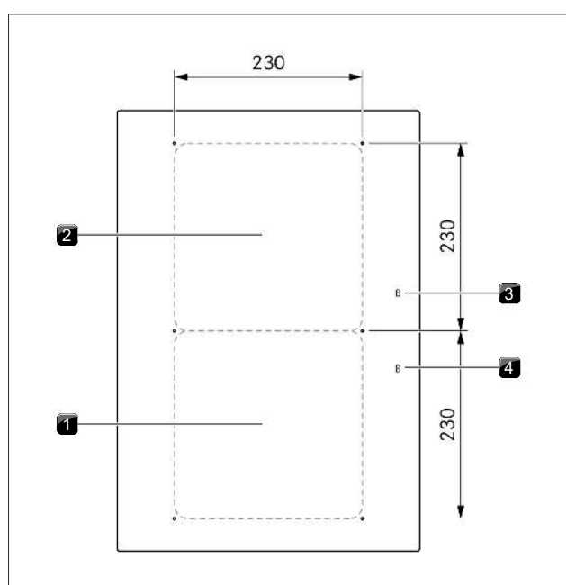
Sl. 3.8 Sestava kuhalne plošče PKFI3/PKFI3R in velikost kuhališč
