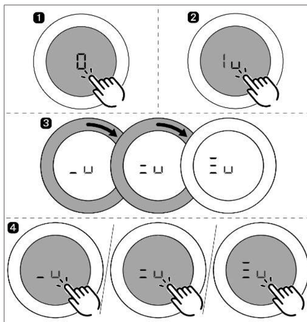
Sl. 5.31 Aktiviranje funkcije za ohranjanje toplote indukcijskih in plinskih kuhalnih plošč
