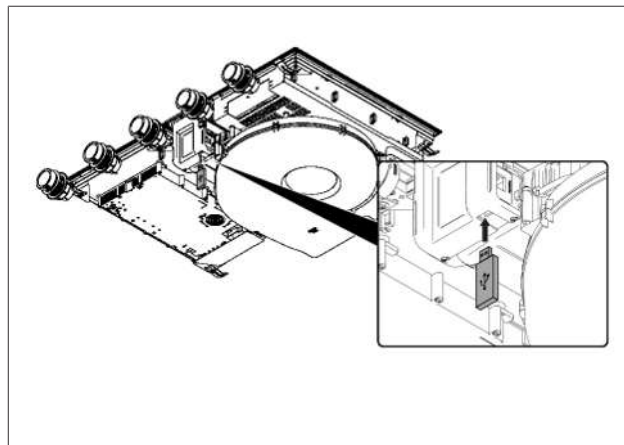
Sl. 6.3 Priklp ključka USB
