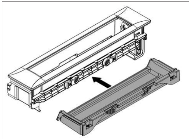
Sl. 7.5 Vgradnja posode za vzdrževanje
